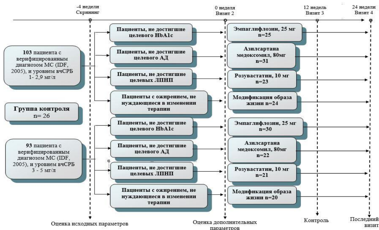
Рисунок 1 - Дизайн исследования.
