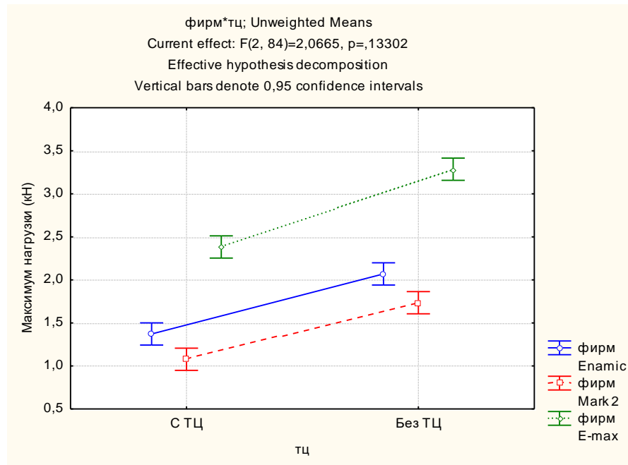
Рисунок 3 – Сравнение максимума нагрузки между группами
