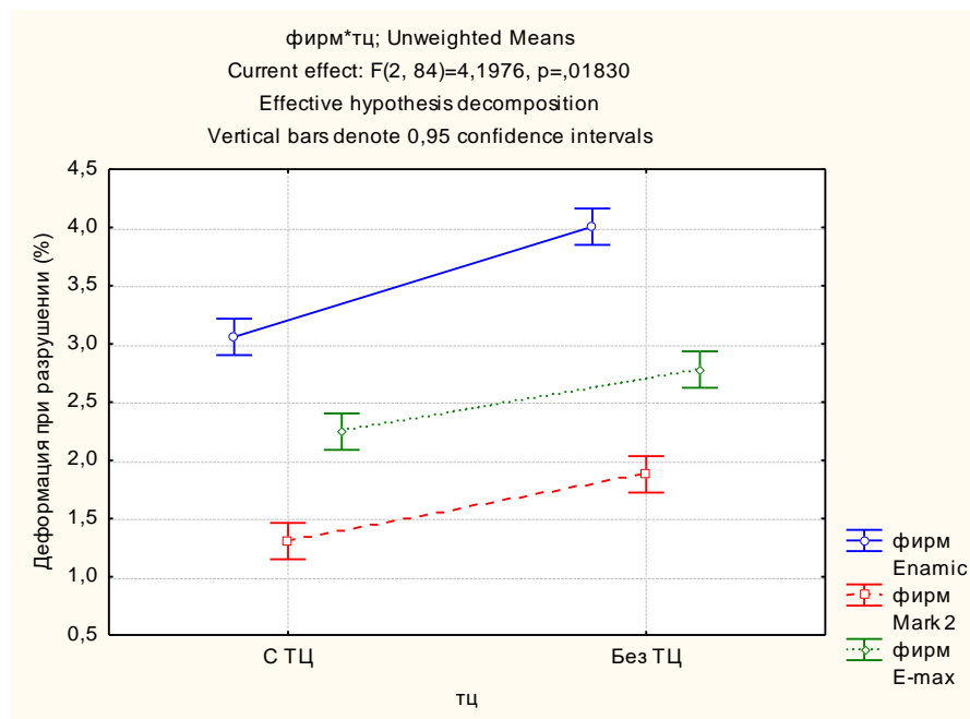
Рисунок 5 – Сравнение максимума деформации при разрушении между группами
