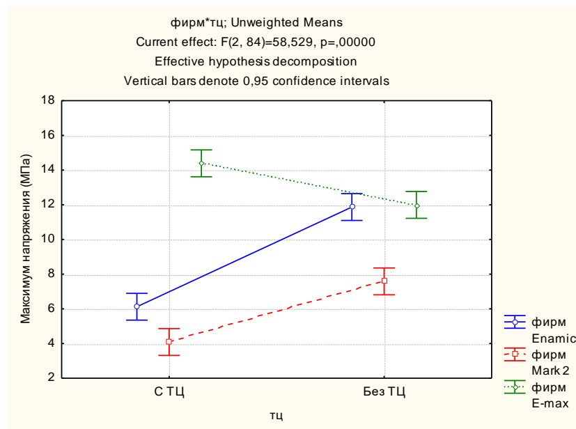
Рисунок 4 – Сравнение максимума напряжения между группами
