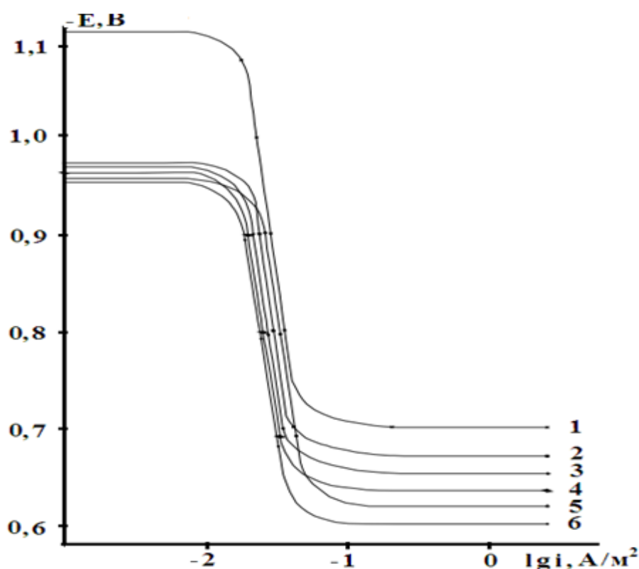
Рисунок 9 – Анодные поляризационные (2мВ/с) кривые алюминиевого сплава Al5Fe10Si (1), содержащего литий, мас.‰: 0.01(2), 0.05(3), 0.1(4), 0.5(5), 1(6), в среде электролита 3.0% - ного NaCl.
