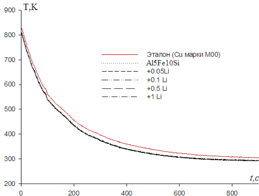
Рисунок 2 – Зависимость температуры образцов от времени охлаждения для образцов из алюминиевого сплава Al5Fe10Si с литием и эталона (Cu марки М00) .
