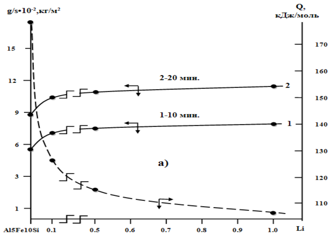
Рисунок 7 – Изохронны окисления алюминиевого сплава \text{Al}_5\text{Fe}_{10}\text{Si} с литием, при температуре 773 К.
