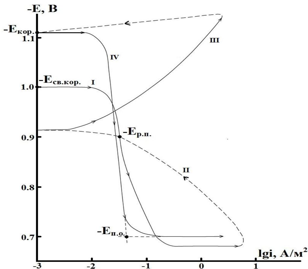
Рисунок 8 – Полная поляризационная (2мВ/с) кривая алюминиевого сплава Al5Fe10Si, в среде электролита 3%-ного NaCl.
