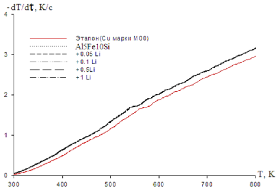
Рисунок 3 – Температурная зависимость скорости охлаждения образцов из сплава Al5Fe10Si с литием и эталона (Cu марки М00).
