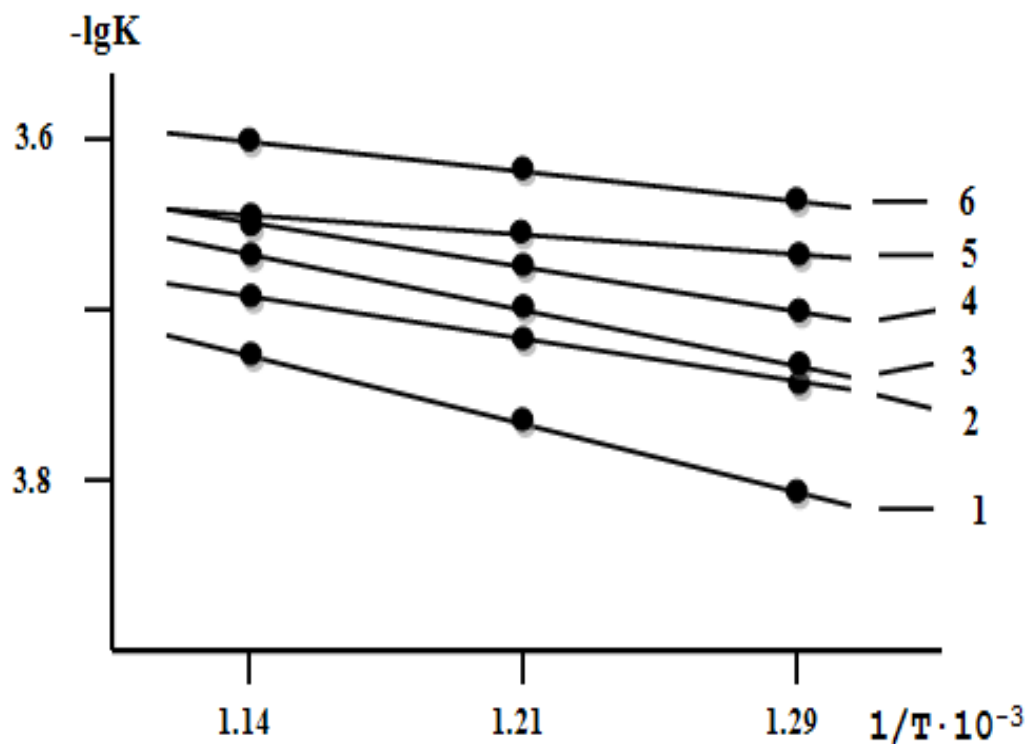
Рисунок 6 – Зависимость \lg K от 1/T для сплава \text{Al}_5\text{Fe}_{10}\text{Si} (1) с литием, мас. % 0,01(2); 0,05(3); 0,1(4); 0,5(5); 1,0(6)
