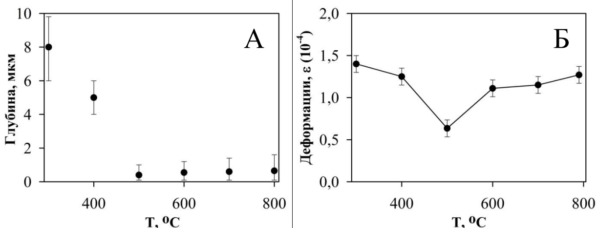
Рис. 7. Зависимость глубины нарушенного приповерхностного слоя (А) и деформации кристаллической решетки НЛ (Б) от температуры предотжига
