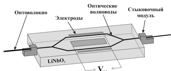
Рис. 2. Схематичное представление ИОС
