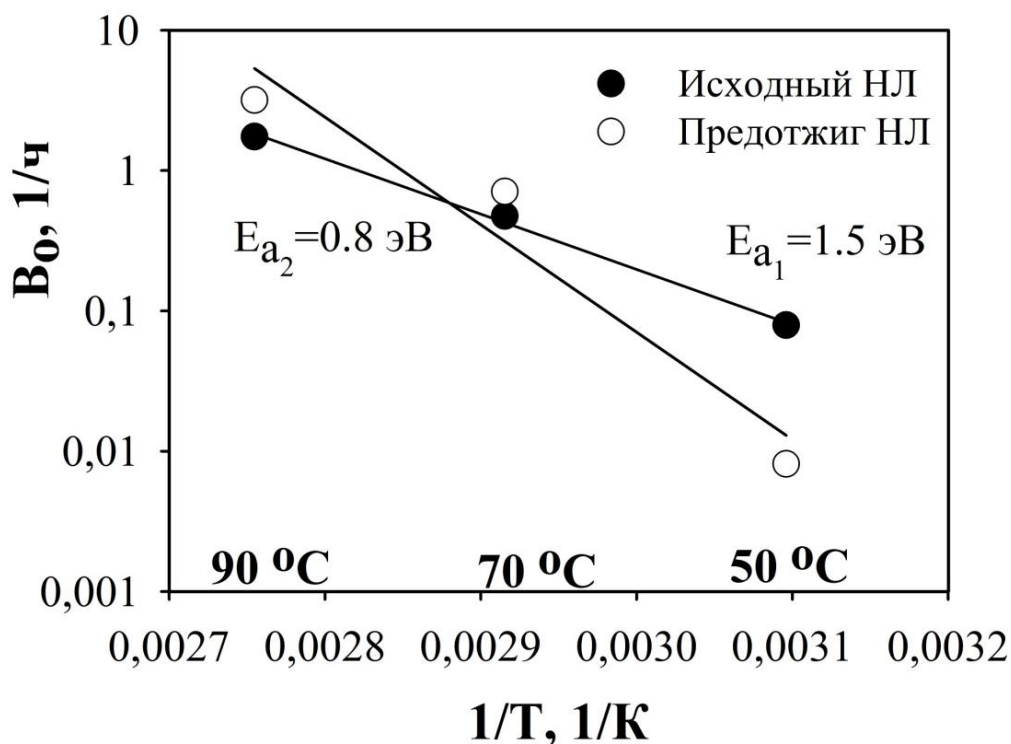
Рис. 10. Графики Аррениуса
