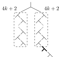
Рисунок 4 — Деревья, длины орбит которых растут как \Theta(n^2)
