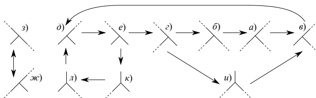
Рисунок 2 — Карусельный эффект для триад
