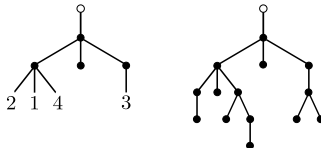
Рисунок 7 — Шаблон дерева
