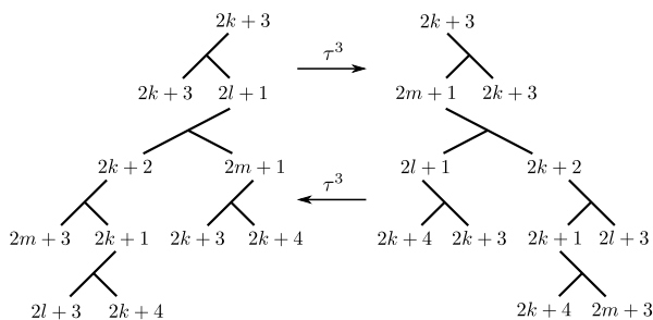
Рисунок 5 — Пример нешапировского цикла
