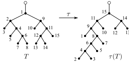
Рисунок 1 — Пример преобразования Донахью
