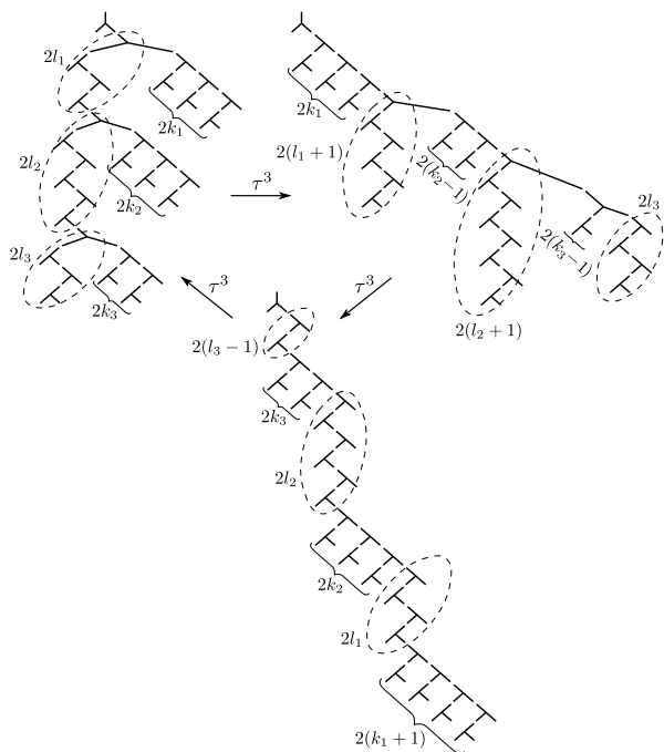
Рисунок 6 — Экспоненциальное семейство циклов длины 9
