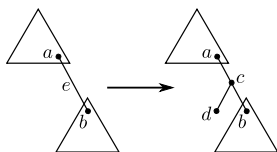
Рисунок 3 — Реализация ростка в дереве
