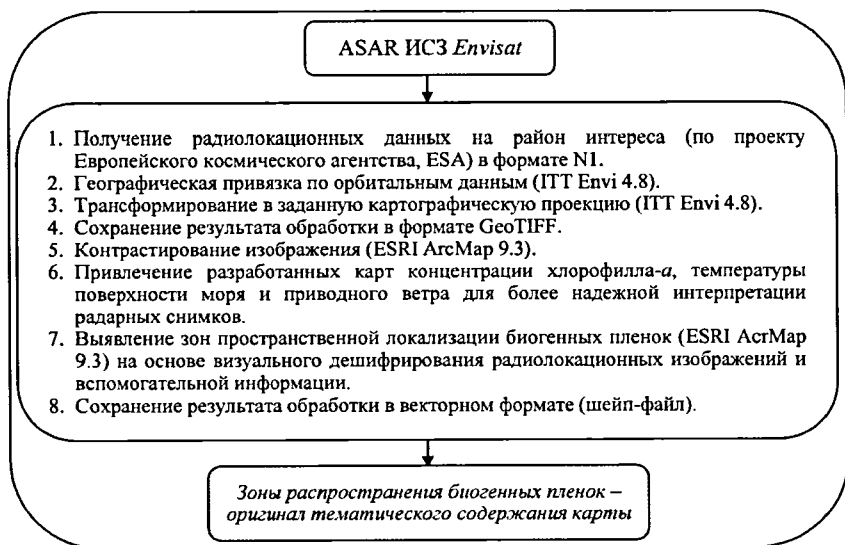
Рис. 4. Технологическая схема обработки данных ASAR ИСЗ Envisat для выявления зон пространственной локализации биогенных пленок.
