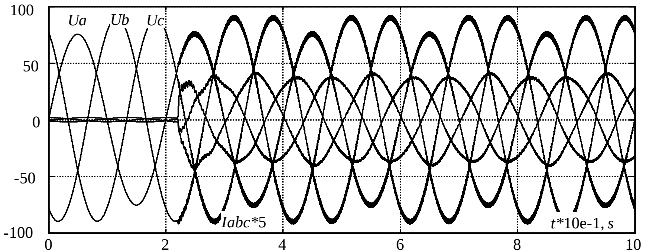
Рисунок 7 – Фазні струми в промисловій мережі при зниженні напруги фази А на 16 % та корекції завдань струмів
