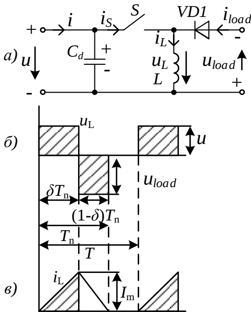
Рисунок 3 – Внутрішня структура інвертуючого ШПП
