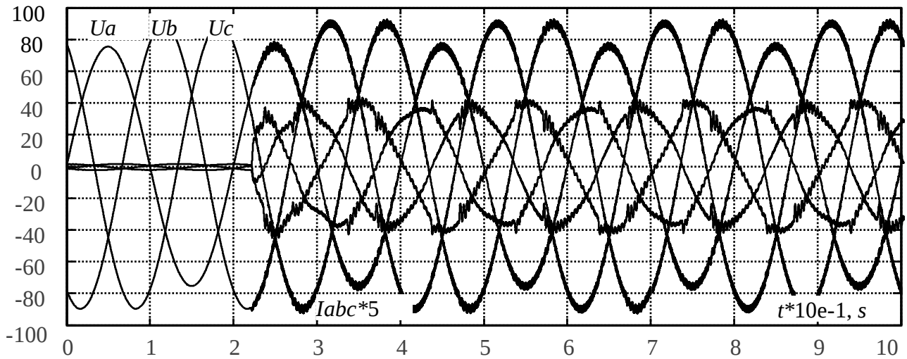
Рисунок 6 – Фазні струми в промисловій мережі при зниженні напруги фази А на 16 %
