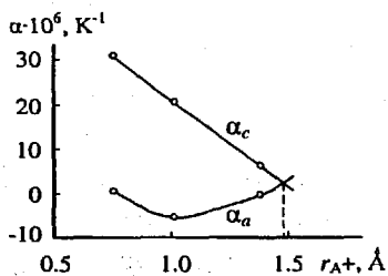
Рис. 12. Термические коэффициенты линейного расширения (298–1073 К) фосфатов ATi_2(PO_4)_3 вдоль осей a и c в зависимости от радиуса катиона A^+
