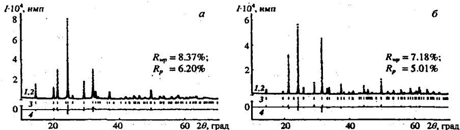
Рис. 2. Фрагменты экспериментальной (1), вычисленной (2), штрих- (3) и разностной (4) дифрактограмм фосфатов \text{Na}_{0.5}\text{K}_{0.5}\text{Ti}_2(\text{PO}_4)_3 (а) и \text{K}_{0.5}\text{Rb}_{0.5}\text{Ti}_2(\text{PO}_4)_3 (б). Экспериментальные дифрактограммы показаны •, вычисленные – сплошной линией.
