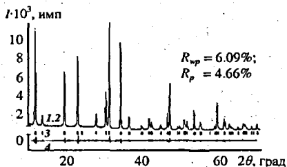
Рис. 10. Фрагмент экспериментальной (1), вычисленной (2), штрих- (3) и разностной (4) дифрактограмм \text{Na}_5\text{Hf}(\text{PO}_4)_3 .
