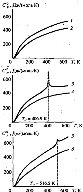
Рис. 13. Температурная зависимость теплоемкости: \text{Na}_5\text{Ti}(\text{PO}_4)_3 (1), \text{NaTi}_2(\text{PO}_4)_3 (2), \text{Na}_5\text{Zr}(\text{PO}_4)_3 (3), \text{NaZr}_2(\text{PO}_4)_3^* (4), \text{Na}_5\text{Hf}(\text{PO}_4)_3 (5), \text{NaHf}_2(\text{PO}_4)_3 (6). (* литературные данные)
