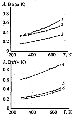
Рис. 14. Температурная зависимость теплопроводности: \text{NaTi}_2(\text{PO}_4)_3 (1), \text{NaZr}_2(\text{PO}_4)_3 (2), \text{NaHf}_2(\text{PO}_4)_3 (3), \text{Na}_5\text{Ti}(\text{PO}_4)_3 (4), \text{Na}_5\text{Zr}(\text{PO}_4)_3 (5), \text{Na}_5\text{Hf}(\text{PO}_4)_3 (6). (относит. плотность 70–80%)
