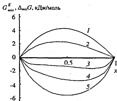
Рис. 17. Концентрационные зависимости избыточной функции Гиббса и функции Гиббса смешения \text{Na}_{1-x}\text{K}_x\text{Ti}_2(\text{PO}_4)_3 (1, 3), \text{Na}_{1-x}\text{K}_x\text{Zr}_2(\text{PO}_4)_3 (2, 4), функции Гиббса смешения идеальных бинарных твердых растворов (5).
