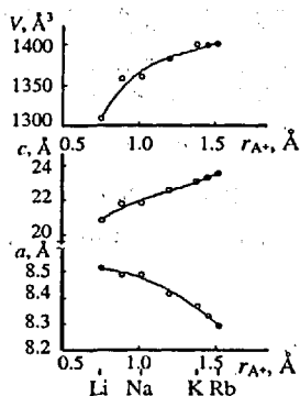
Рис. 4. Изменение параметров ячеек \text{ATi}_2(\text{PO}_4)_3 и тройных \text{A}_{0.5}\text{A}'_{0.5}\text{Ti}_2(\text{PO}_4)_3 фосфатов в зависимости от радиуса катионов щелочных металлов.
