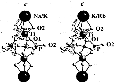
Рис. 5. Деформации структурных фрагментов каркаса в зависимости от радиуса катионов щелочных металлов во внекаркасных позициях M1: \text{Na}_{0.5}\text{K}_{0.5}\text{Ti}_2(\text{PO}_4)_3 (а), \text{K}_{0.5}\text{Rb}_{0.5}\text{Ti}_2(\text{PO}_4)_3 (б).
