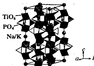
Рис. 3. Структура \text{Na}_{0.5}\text{K}_{0.5}\text{Ti}_2(\text{PO}_4)_3
