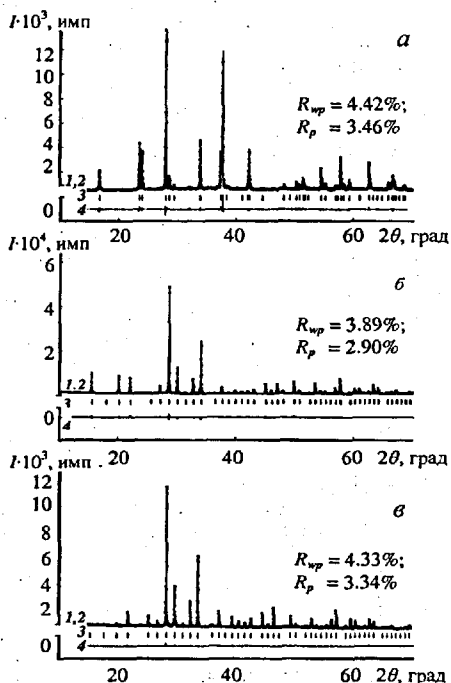
Рис 7. Фрагменты экспериментальной (1) вычисленной (2), штрих- (3) и разностной (4) дифрактограмм \text{Na}_2\text{FeTi}(\text{PO}_4)_3 (а), \text{K}_2\text{FeTi}(\text{PO}_4)_3 (б) и \text{Rb}_2\text{FeTi}(\text{PO}_4)_3 (в).
