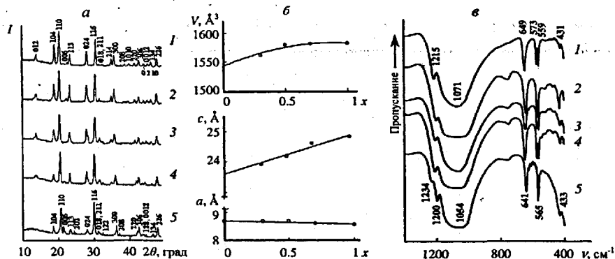
Рис. 1. Дифрактограммы (а), параметры элементарных ячеек (б) и ИК-спектры (в) фосфатов \text{K}_{1-x}\text{Cs}_x\text{Hf}_2(\text{PO}_4)_3 : x = 0 (1), 0.3 (2), 0.5 (3), 0.7 (4), 1.0 (5).
