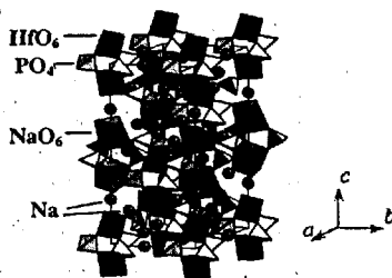
Рис. 11. Структура \text{Na}_5\text{Hf}(\text{PO}_4)_3 .
