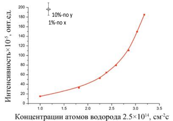
Рисунок 12. Интенсивность ГХЛ Н ZnS–Eu в зависимости от плотности потока возбуждающих атомов водорода. Температура 295 K
