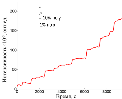
Рисунок 11. Приращение интенсивности ГХЛ Н ZnS–Eu при ступенчатом увеличении концентрации атомов водорода. T = 295 K, давление H+H_2 в разрядной трубке 3.0 \cdot 10^{-2} торр. Образец предварительно прогрет 30 минут в вакууме при 473K.
