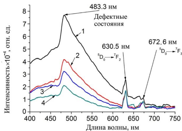
Рисунок 13. Спектр фотолюминесценции AlN-Eu 3+ при возбуждении ртутной лампой ДРТ 125-1 с фильтром УФС-06 (317-340 нм): 1 – 305 К, 2 – 400 К, 3 – 457 К, 4 – 493 К.
