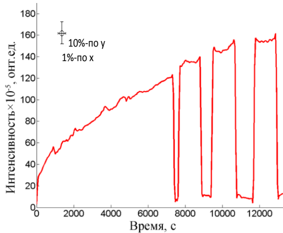
Рисунок 10 Интенсивность ГХЛ Н люминофора ZnS–Eu при «выключении» и «включении» атомов водорода – «темновые» паузы. Температура образца 306K, давление в разрядной трубке 3.0 \cdot 10^{-2} торр. Образец предварительно прогрет в вакууме при 473K , 30 мин.
