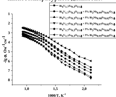
Рисунок 7 – Температурная зависимость электропроводности образцов \text{Bi}_4\text{V}_{1.7}\text{Fe}_{0.3}\text{O}_{11-\delta} / 5% \text{Bi}_3\text{Nb}_{1-y}\text{Fe}_y\text{O}_{7-\delta}
