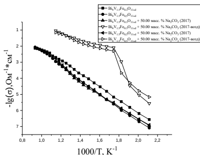
Рисунок 19 – Температурные зависимости электропроводности смесей BIFEVOX с Na 2 CO 3 : а) с петлей гистерезиса, б) с выдержкой в атмосфере окружающей среды
