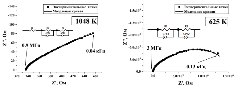
Рисунок 4 – Типичные диаграммы импеданса для \text{Bi}_4\text{V}_{1.5}\text{Fe}_{0.5}\text{O}_{11-\delta} + 50\% \text{Bi}_2\text{O}_3 при 1048 и 625 K
