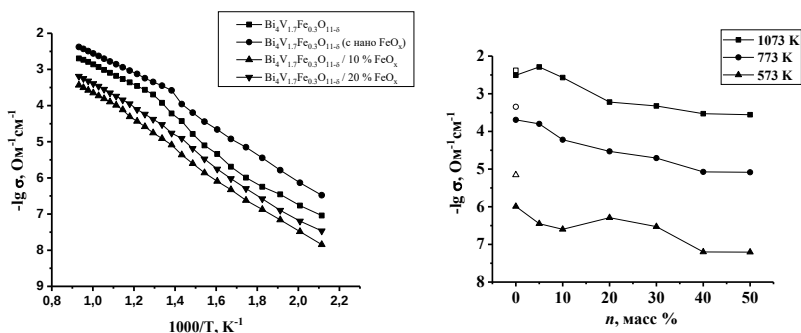
Рисунок 12 – Температурная и концентрационная зависимости электропроводности серии композитов состава \text{Bi}_4\text{V}_{1.7}\text{Fe}_{0.3}\text{O}_{11-\delta} / n \text{FeO}_x (открытые значки относятся к \text{Bi}_4\text{V}_{1.7}\text{Fe}_{0.3}\text{O}_{11-\delta} в ходе получения которого использовался нано- \text{FeO}_x )
