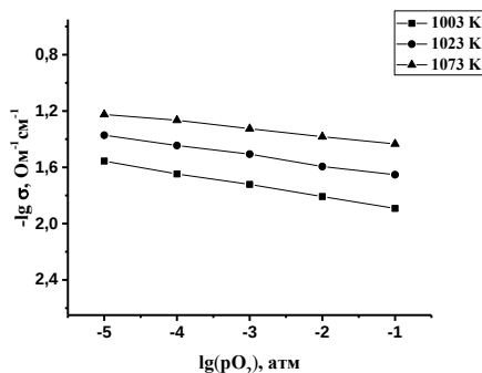
Рисунок 6 – Зависимость электропроводности твёрдого раствора состава \text{Bi}_4\text{V}_{1.7}\text{Fe}_{0.3}\text{O}_{11-\delta} / 2.5 % \text{Bi}_2\text{O}_3 от парциального давления кислорода
