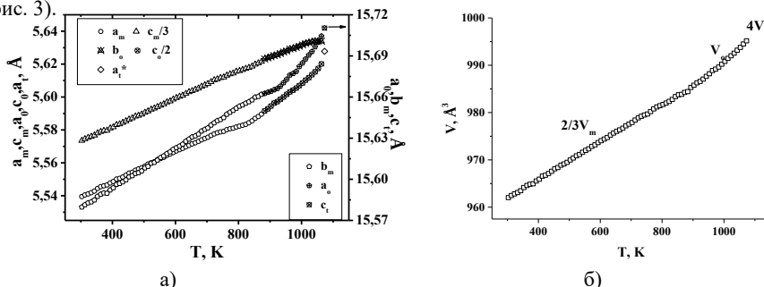
Рисунок 3 – Температурная зависимость ПЭЯ (а) и объема (б) образца \text{Bi}_4\text{V}_{1.5}\text{Fe}_{0.5}\text{O}_{11-\delta} / 20 % \text{Bi}_2\text{O}_3 в температурном интервале 303 – 1073 К
