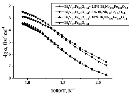
Рисунок 8 – Температурная зависимость электропроводности образцов \text{Bi}_4\text{V}_{1.7}\text{Fe}_{0.3}\text{O}_{11-\delta} / n \text{ Bi}_3\text{Nb}_{0.96}\text{Fe}_{0.04}\text{O}_{7-\delta}
