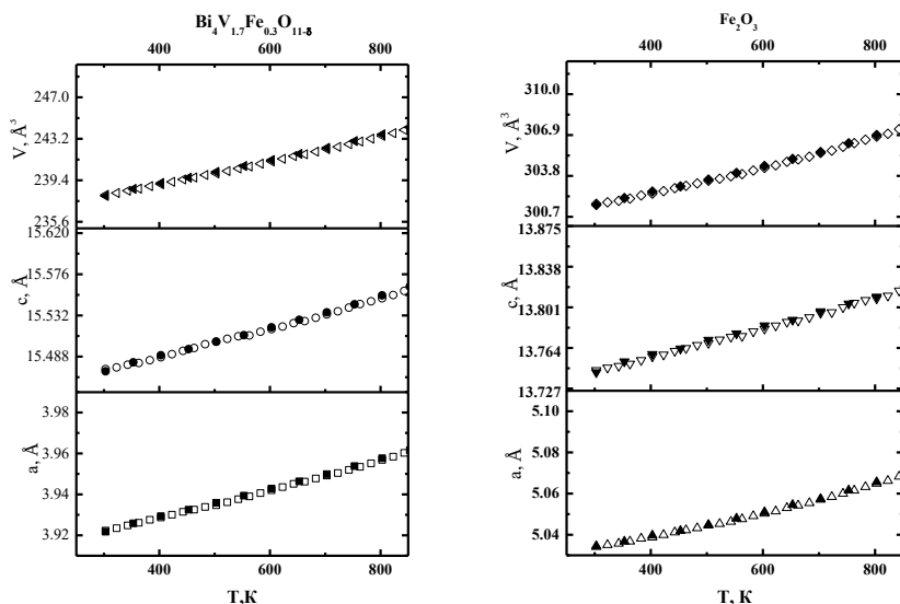
Рисунок 10 – Температурная зависимость ПЭЯ сосуществующих фаз в образце \text{Bi}_4\text{V}_{1.7}\text{Fe}_{0.3}\text{O}_{11.8}/50\% \text{FeO}_x в температурном интервале 303 – 1073 К. Пустые символы – нагревание, заполненные – охлаждение.
