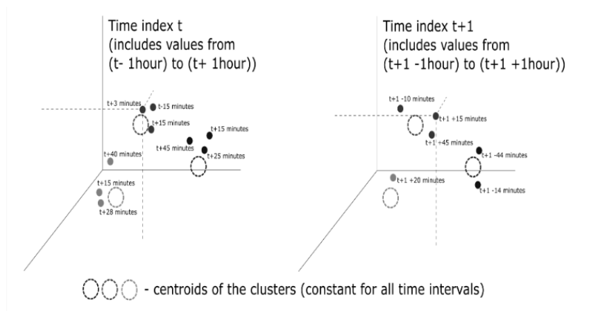
Рисунок 4 – Первый этап работы программы, на котором выбирается временной шаг дискретизации пространства сейсмических событий
