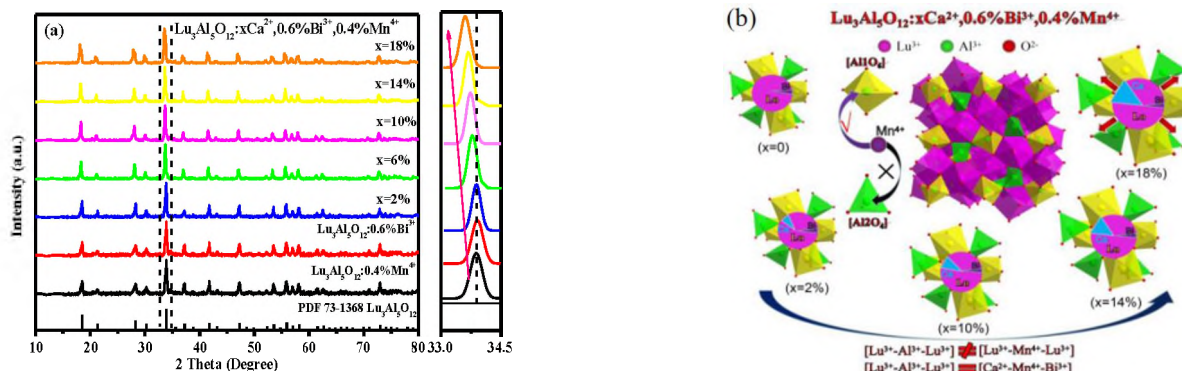
Рисунок 7 - Рентгенограмма люминофоров Lu_3Al_5O_{12}:0.4\%Mn^{4+} , Lu_3Al_5O_{12}:0.6\%Bi^{3+} и Lu_3Al_5O_{12}:xCa^{2+}, 0.6\%Bi^{3+}, 0.4\%Mn^{4+} при различных значениях x (а) (справа - увеличенная рентгенограмма между 2\theta и 33.0^\circ - 34.5^\circ ) и схематическое изображение механизма замещения ионов при легировании и влияния Ca^{2+} на локальные кристаллические структуры (б).
