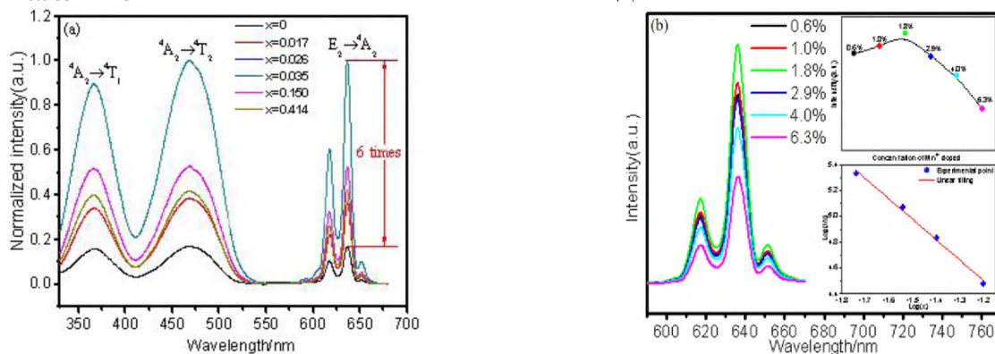
Рисунок 3 – Спектры ФЛВ и ФЛ (25°C) \text{BaTiF}_6:0.6\%\text{Mn}^{4+} и \text{K}_{2x}\text{Ba}_{1-x}\text{TiF}_6:1.8\%\text{Mn}^{4+} в зависимости от значения x (а) (на вставке показан цвет \text{BaTiF}_6:0.6\%\text{Mn}^{4+} и \text{K}_{0.070}\text{Ba}_{0.965}\text{TiF}_6:1.8\%\text{Mn}^{4+} при естественном освещении и при облучении УФ-лампой) и спектры ФЛ \text{K}_{0.070}\text{Ba}_{0.965}\text{TiF}_6:y\text{Mn}^{4+} при разных значениях y (б).
