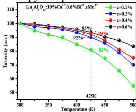
Рисунок 10 - Температурная зависимость интегрированной интенсивности излучения \text{Lu}_3\text{Al}_5\text{O}_{12}:10\%\text{Ca}^{2+}, 0.6\%\text{Bi}^{3+}, z\text{Mn}^{4+} в зависимости от концентрации z ионов \text{Mn}^{4+}
