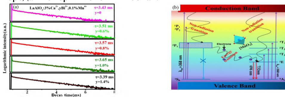
Рисунок 14 - Кинетика затухания люминесценции люминофоров \text{LaAlO}_3:3\%\text{Ca}^{2+}, y\text{Bi}^{3+}, 0.1\%\text{Mn}^{4+} ( y=0, 0.6\%, 0.8\%, 1.0\% и 1.4\% ) при возбуждении при 368 нм и мониторинге при 732 нм (а) и схема передачи энергии от \text{Bi}^{3+} до \text{Mn}^{4+} (б).
