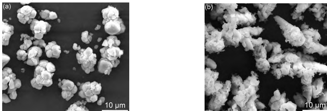
Рисунок 2 - SEM-изображение образца BaTiF_6:0.6\%Mn^{4+} (а) и SEM-изображение образца K_{0,070}Ba_{0,965}TiF_6:1.8\%Mn^{4+} (б).
