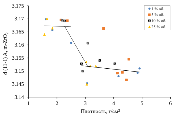
Рисунок 7. Зависимость межплоскостного расстояния d_{11-1} A, m-ZrO 2 от плотности
