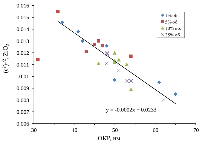
Рисунок 9. Зависимость микродеформации (\epsilon^2)^{1/2} от ОКР моноклинного диоксида циркония в спеченных композитах
