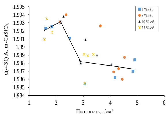
Рисунок 8. Зависимость межплоскостного расстояния d_{-431} A, m-CaSiO 3 от плотности
