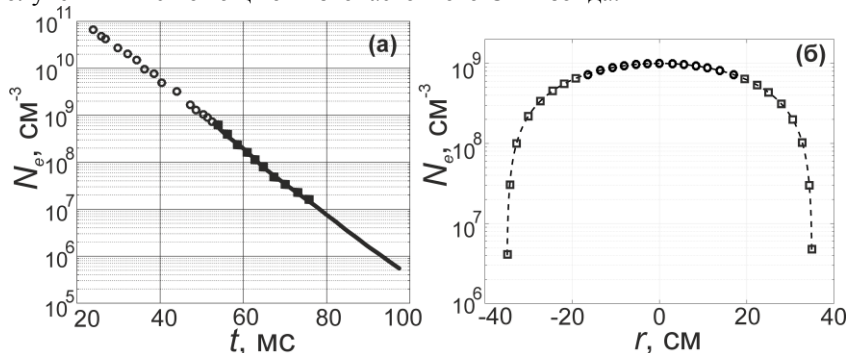
Рис. 2. (а) Временная зависимость концентрации плазмы после окончания работы плазмосоздающего источника: сплошная кривая – измерения выполнены малогабаритным СВЧ-зондом ( f_0 = 2034 МГц) с применением амплитудно-фазовой методики, \circ – измерения выполнены тем же использованием стандартной методики, \square – измерения выполнены низкочастотным СВЧ-зондом ( f_0 = 420 МГц) с использованием стандартной методики. (б) Радиальное распределение концентрации плазмы на стенде «Ионосфера» в момент времени t = 50 мс после пробоя плазмы. Измерения проводились малогабаритным СВЧ-зондом ( f_0 = 2034 МГц): \circ – измерения выполнены с использованием стандартной методики, \square – измерения выполнены при помощи амплитудно-фазового метода.
