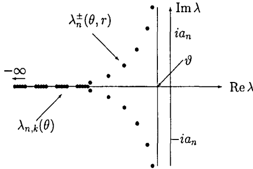
Рис. 4: Структура спектра в случае K(t) \in L_1(\mathbb{R}_+) , но K(t) \notin W_1^1(\mathbb{R}_+) .
