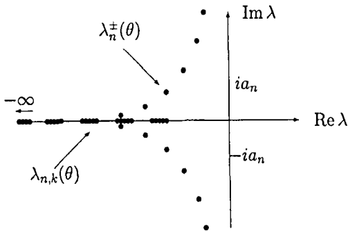
Рис. 1: Структура спектра в случае, когда K(t) \in W_1^1(\mathbb{R}_+) .
