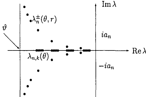
Рис. 5: Структура спектра в случае K(t) \in L_1(\mathbb{R}_+) , но K(t) \notin W_1^1(\mathbb{R}_+) .
