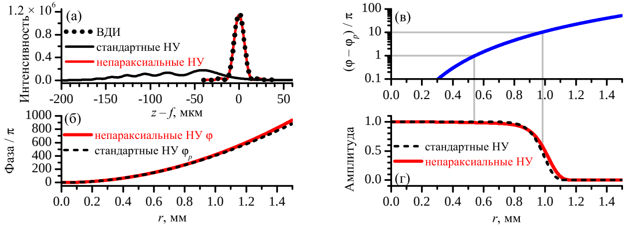
Рис. 2 — Фокусировка параболическим зеркалом f = 3 мм ( f/1.5 , NA = 0.33 ). (а) Зависимость |E_x|^2(x = y = 0, z) , рассчитанная со стандартными (черная кривая) и непараксиальными (красная кривая) начальными условиями, а также с помощью ВДИ (черные точки). (б) Фаза и (г) амплитуда стандартных (черный пунктир) и непараксиальных (красная кривая) начальных условий. Рисунок (в) показывает разницу между фазами (б).
