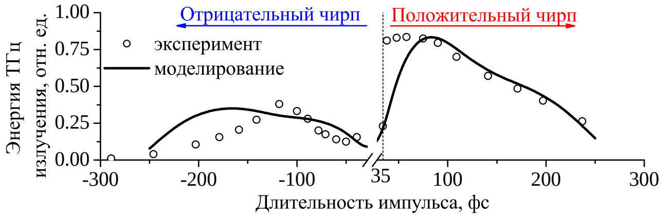
Рис. 8 — Зависимость энергии ТГц излучения двуцветного филамента от длительности чирпированного импульса. Эксперимент проведен в группе проф. Y. Chen (Shanghai Jiao Tong Univ., Шанхай, Китай) [A3].
