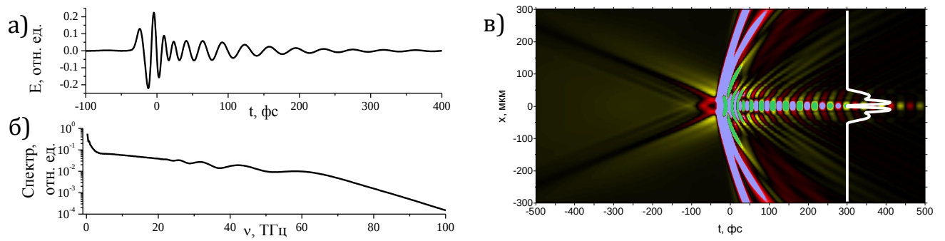
Рис. 11 — (а) Волновая форма, (б) интегральный спектр и (в) (x, t) -распределение терагерцового поля при филаментации двуцветного излучения, регуляризованного четырехсекционной фазовой пластинкой. Белая кривая справа изображает поперечный профиль плазмы.
