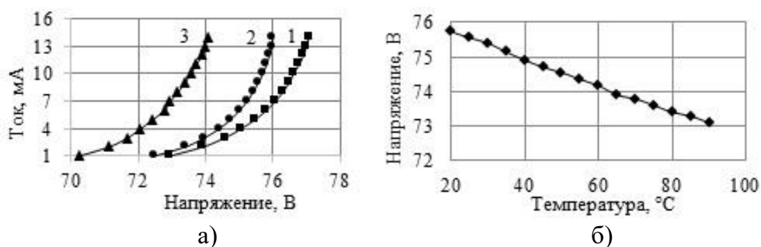
Рисунок 12 – ВАХ при разных значениях температуры (а) и температурная зависимость напряжения при значении прямого тока 10 мА (б).
