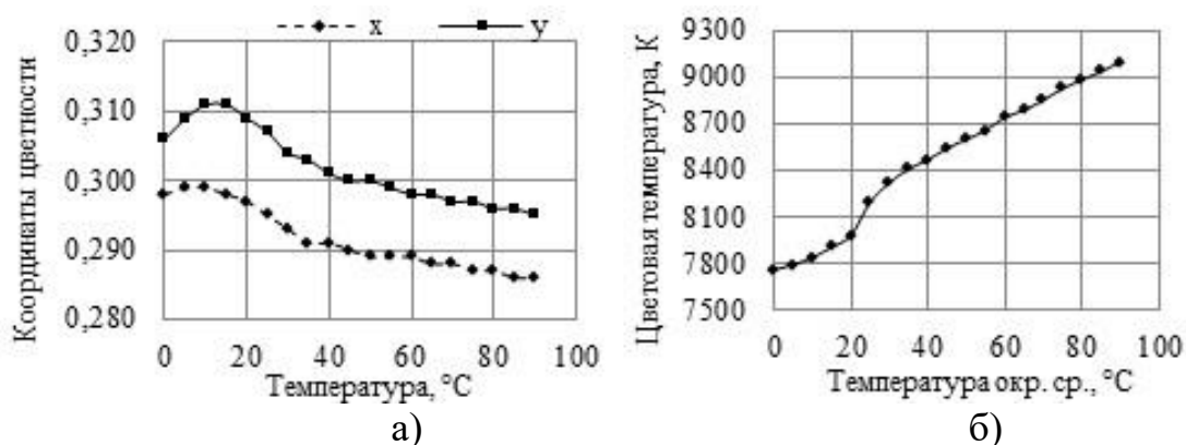
Рисунок 13 – Зависимость цветовых координат (а) и коррелированной цветовой температуры (б) от температуры окружающей среды.
