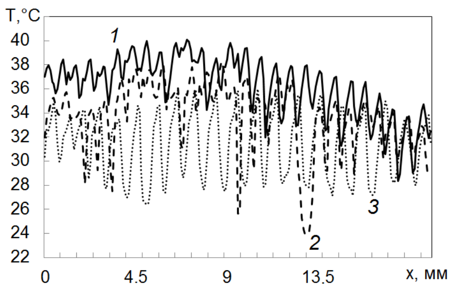
Рисунок 10 – Сравнение температурных профилей с локализацией кристаллов: Кривая 1 – I = 5 мА, Coeff = 1,0 ; кривая 2 – I = 5 мА, Coeff = 1,0 ; кривая 3 – I = 5 мА, Coeff = 1,5 .
