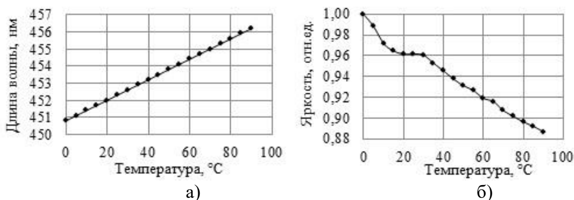
Рисунок 14 – Температурная зависимость доминирующей длины волны (а) и температурная зависимость яркости (б) при значении прямого тока 10 мА.
