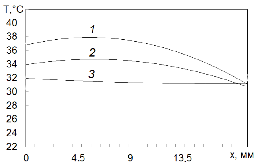
Рисунок 11 – Результат аппроксимации графиков на рисунке 8.
