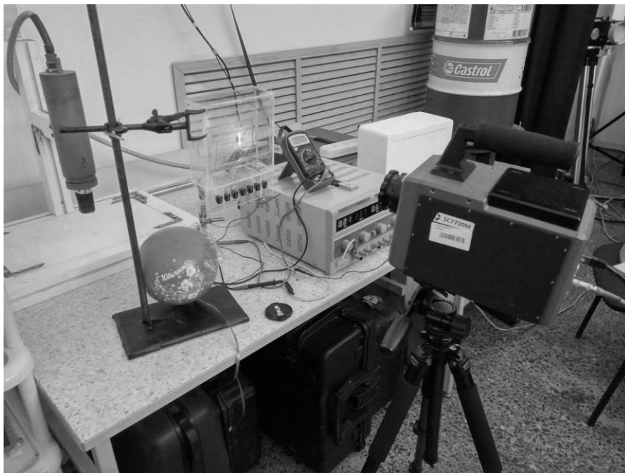
Рисунок 7 – Внешний вид измерительной установки
