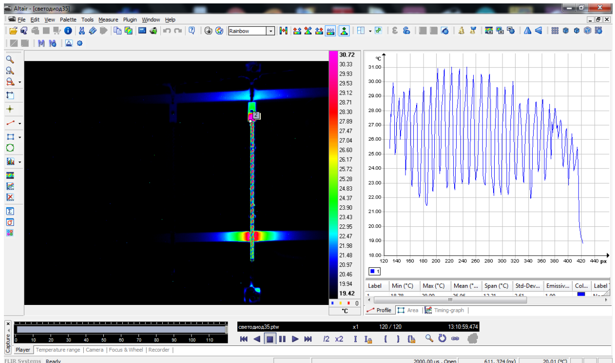
Рисунок 9 – Температурный профиль ФСНМ без люминофорного покрытия
