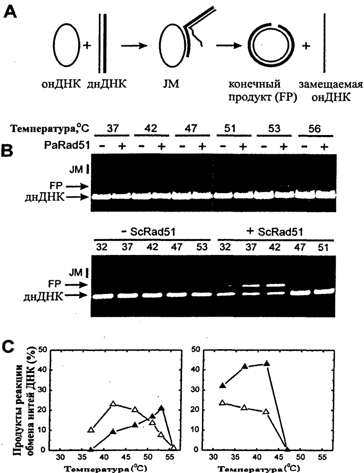
Рис. 1. Реакция переноса нити in vitro , катализируемая белками Rad51 Pa (PaRad51) или Rad51 Sc (ScRad51) зависит от температурных условий. (А) Схема реакции обмена нити ДНК между \phi X174 онДНК (плюс нить) и репликативной формой линейной днДНК того же фага. (В) Тестирование реакции обмена нити ДНК в агарозном гель-электрофорезе. JM (joint molecules) – связанная молекула ДНК, промежуточный продукт реакции переноса нити; FP (final products) – конечные продукты переноса нити ДНК. (С) Графическое представление относительных количества JM и FP, определенных из теста (В) (см. Материалы и методы). Обозначения: белый треугольник, JM; черный треугольник, FP. Слева, Rad51 Pa ; справа, Rad51 Sc .
