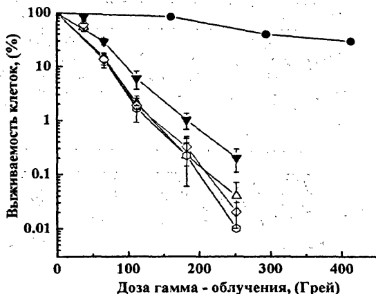
Рис. 2. Чувствительность клеток дрожжей S. cerevisiae к действию \gamma -излучения в жидкой среде. Обозначения: Диплоидный штамм ( rad51/rad51 ), трансформированный плазмидой pYES2::RAD51 Pa , несущей ген RAD51 из P. angusta под контролем регулируемого промотора GAL1 : на среде без индуктора (—○—); на среде с индуктором (—▼—). Диплоидный штамм ( rad51/rad51 ), трансформированный плазмидой pYES2: на среде без индуктора (—○—); на среде с индуктором (—○—). Диплоидный штамм дикого типа (Wt 2n RAD+) (—●—). Стандартное отклонение ( \pm ) определялось из трех экспериментов.
