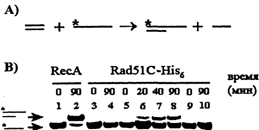
Рис. 4. Радиоавтограф электрофореграммы реакции переноса нитей ДНК. А) Схема тестирования ДНК-трансферазной активности с использованием радиоактивномеченного ДНК-субстрата. В) Кинетика реакции переноса нити ДНК с радиоактивномеченным субстратом. Дорожки 1, 2 - реакция с белком RecA в течение 0 и 90 минут, соответственно. Дорожки 3, 4 - контрольная реакция с белком Rad51C C -His 6 , когда в реакции отсутствует гомологичная днДНК в течение 0, 90 минут, соответственно. Дорожки 5, 6, 7, 8 - реакция с белком Rad51C C -His 6 и гомологичными ДНК-субстратами в течение 0, 20, 40, и 90 минут, соответственно. Дорожки 9, 10 - контрольная реакция с белком Rad51C C -His 6 , когда в реакции присутствует гетерологичная, в течение 0, 90 минут, соответственно.
