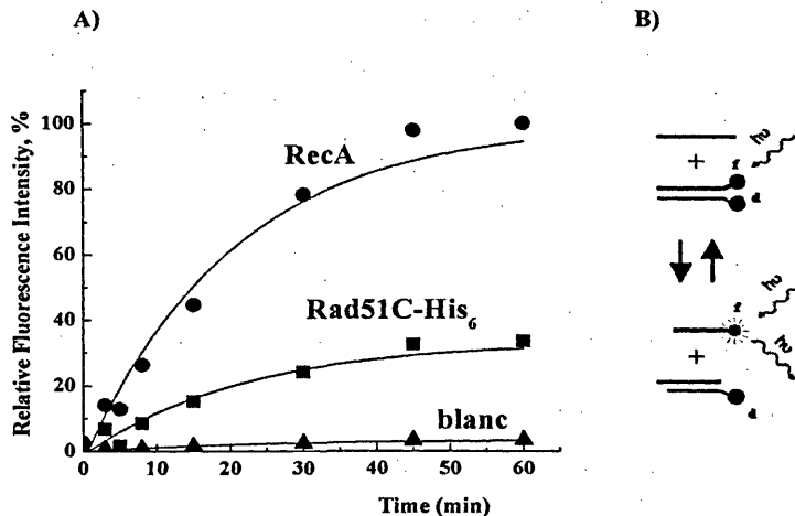
Рис. 3. Кинетика реакции замещения нити ДНК с использованием флуоресцентномеченных субстратов (см. Материалы и методы). А) Реакция замещения нити ДНК для белков RecA и Rad51C Q -His 6 в присутствии ATP; В) схема реакции замещения нити ДНК.
