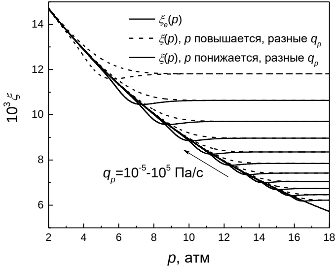
Рис. 13. Зависимость структурного параметра системы от давления, \zeta = \zeta(p) , при переходе жидкость-стекло для разных значений скорости изменения давления в интервале 10^{-5} \leq |q_p| \leq 10^5 Па/с. Пунктирные кривые – рост давления, сплошные – уменьшение давления.
