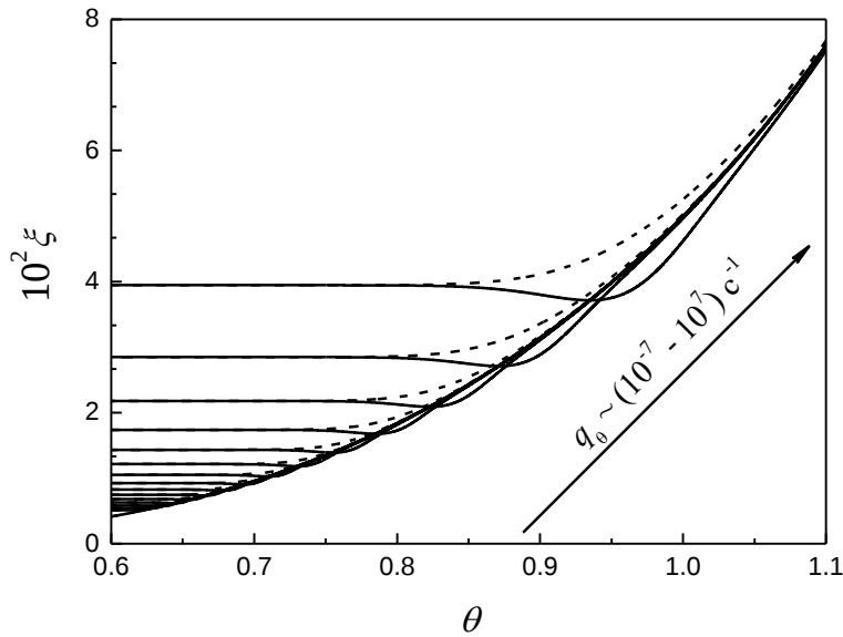
Рис. 12. Зависимость \xi=\xi(\theta) при стекловании модельной системы для разных значений скорости охлаждения (пунктирные кривые) и нагрева (сплошные кривые) в диапазоне 10^{-7} \text{ c}^{-1} \leq q_0 \leq 10^7 \text{ c}^{-1} .
