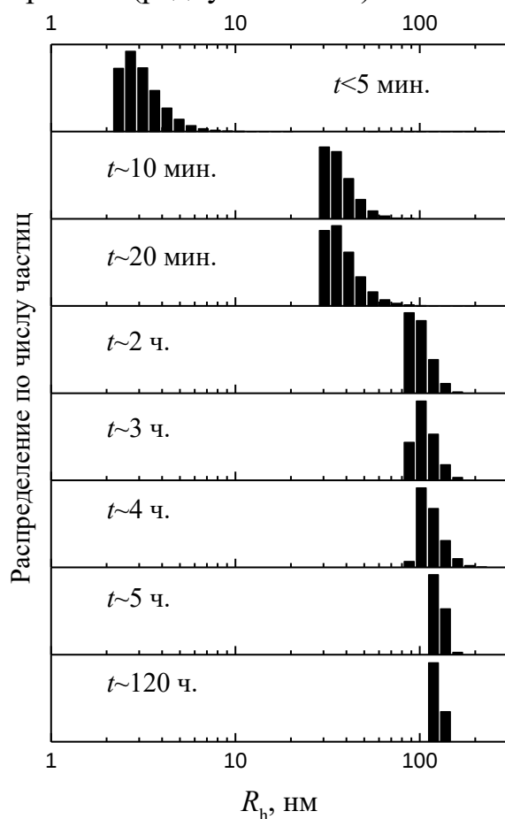
Рис. 3. Эволюция распределения частиц по размерам в растворе C_{60} /НМП по данным метода ДРС.
