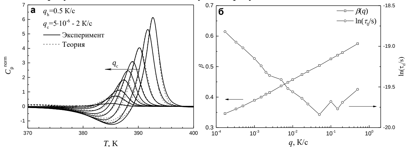
Рис. 9. а - Сравнение экспериментальных и модельных кривых зависимости теплоемкости полистирола от температуры в интервале стеклования. Сплошные кривые – эксперимент, пунктирные – моделирование. Значения параметров A/R , T_0 и \chi соответствуют выражению ФФТ для зависимости T_g(q) , значения параметров \ln\tau_0 и \beta изменяются для каждой скорости охлаждения образца q (б).
