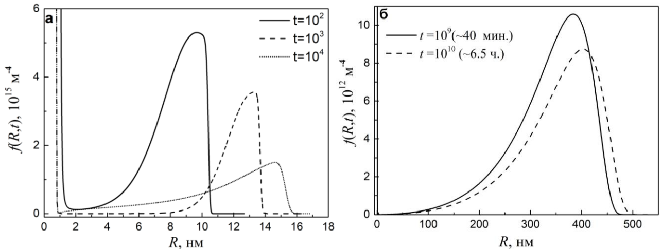
Рис. 5. Рассчитанные функции распределения кластеров C_{60} по размерам в модельном полярном растворе. а – начальные стадии роста кластеров (время менее 1 с); б – рост крупных кластеров, время эволюции системы указано на рисунке.
