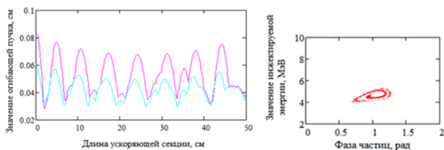
Рисунок 2 – Огибающая пучка и фазовый портрет частиц
