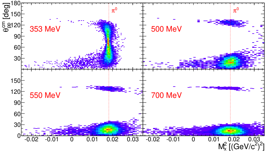
Рис. 4 — Двумерное распределение полярного угла ^1S_0 дипротона в системе центра масс реакции \theta_{pp}^{\text{cm}} относительно квадрата недостающей массы M_X^2 для событий pp \rightarrow \{pp\}_s X .
