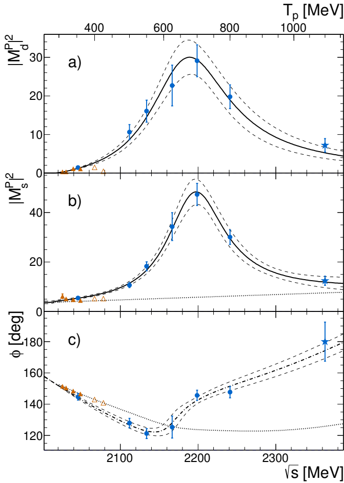
Рис. 8 — Энергетические зависимости квадратов амплитуд для переходов ^3P_2 \rightarrow ^1S_0d (a), ^3P_0 \rightarrow ^1S_0s (b) и их относительной фазы \phi (c). Сплошными линиями показано описание значений |M_d^P|^2 (a) и |M_s^P|^2 модифицированными формами Брейта-Вигнера (b). Штрихпунктирная линия на (c) показывает описание значений \phi эмпирической зависимостью. Диапазоны, обозначенные штриховой линией, показывают интервал 68% достоверности. Обозначения экспериментальных точек аналогичны рис. 7. Звёзды при энергии пучка T_p = 1100 МэВ соответствуют результатам фита с использованием сечения d\sigma/d\Omega и экстраполяции |M_d^P|^2 . Незаполненные треугольники исключены из фита по причинам, описанным в тексте. Источники ошибок те же, что на рис. 7. Пунктирная линия в (b) обозначает фон зависимости Брейта-Вигнера. Пунктирная линия в (c) показывает относительную фазу амплитуд ^3P_0 и ^3P_2 упругого pp \rightarrow pp рассеяния.
