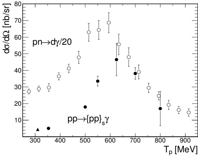
Рис. 10 — Энергетические зависимости дифференциального сечения реакций pp \rightarrow \{pp\}_s \gamma и pn \rightarrow d \gamma . Чёрные кружки соответствуют данным ANKE-COSY для усреднённого дифференциального сечения d\sigma/d\Omega_{(0-20)} реакции pp \rightarrow \{pp\}_s \gamma , в то время как треугольник иллюстрирует результаты CELSIUS [74; 75] для тех же условий по E_{pp} и углам. Пустые окружности показывают значения дифференциального сечения реакции pn \rightarrow d \gamma для угла дейтрона в СЦМ \theta_d = 20^\circ , измеренного относительно импульса протона, которые были получены из данных фоторасщепления дейтрона по работе [28] и отмасштабированы в двадцать раз.
