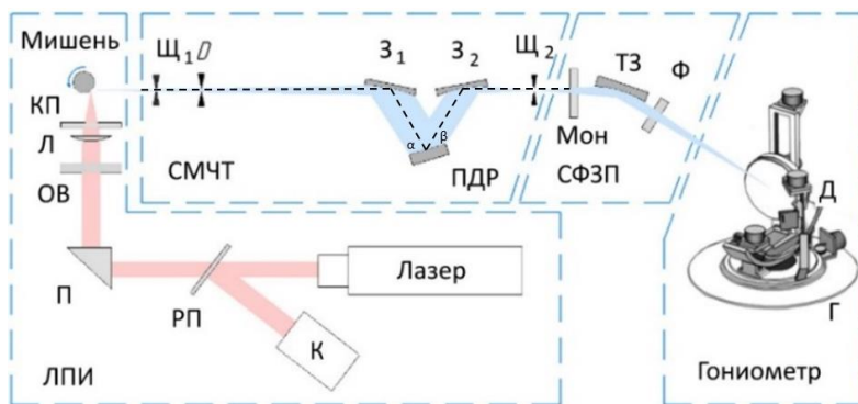
Рис. 3. Оптическая схема рефлектометра
