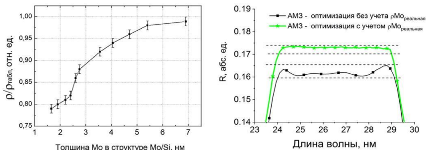
Рис. 1. Слева - зависимость плотности Мо от толщины слоя в ПМЗ Мо/Si; справа - оптимизированные профили коэффициента отражения АМЗ Мо/Si с учетом реальных значений плотности Мо (звездочки) и без (квадраты).
