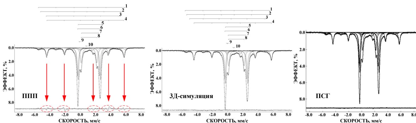
Рисунок 1 – Мессбауэровский спектр фрагмента No 1a метеорита Челябинск LL5, аппроксимированный с использованием трех методов описания компоненты троилита (приведены компоненты, полученные в результате наилучшей аппроксимации, детальное описание приводится в главе 3). Дифференциальные спектры приведены под мессбауэровскими спектрами. Стрелками и пунктирными линиями на дифференциальном спектре показаны ошибки в результате некорректной аппроксимации компоненты троилита методом ППП.
