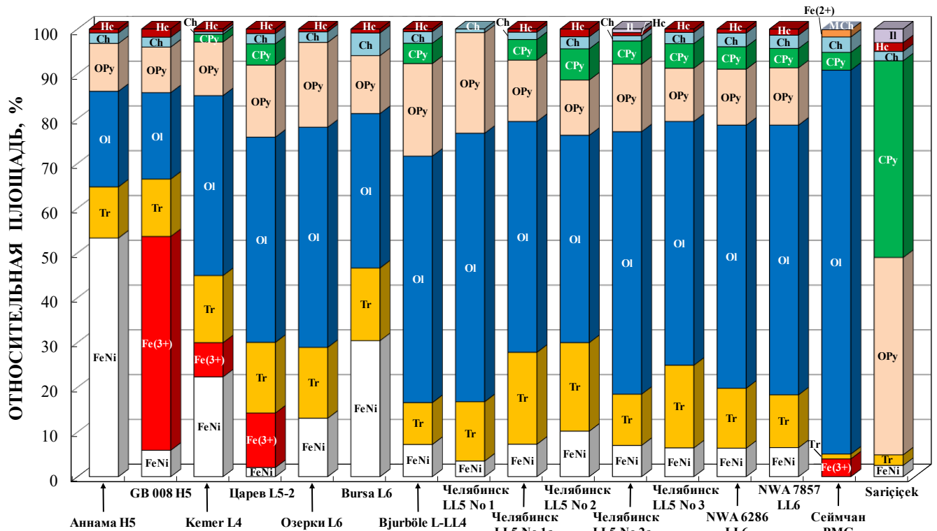
Рисунок 3 – Гистограммы относительных площадей компонент мессбауэровских спектров исследуемых недифференцированных и дифференцированных метеоритов. Обозначения: GB 008 H5 – Gandom Beryan 008 H5, FeNi – сплав Fe-Ni-Co, Fe(3+) – соединения \text{Fe}^{3+} (продукты окисления в результате земного выветривания), Tr – троилит, Ol – оливин, Op – ортопироксен, Cp – клинопироксен, Ch – хромит, Hc – герцинит, Fe(2+) – соединения \text{Fe}^{2+} , Il – ильменит, MCh – магнезиохромит.
