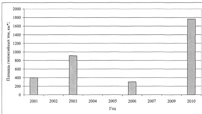
Рисунок 1 – Межгодовая изменчивость площади гипоксических зон в восточной части Финского залива
