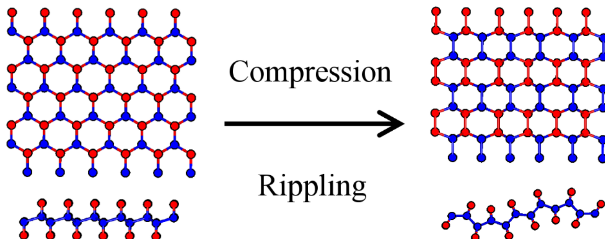
Рисунок 9. Сжатие полностью функционализированного графена приводит к его искривлению и меняет наиболее энергетически выгодный способ упорядочения функциональных групп на его поверхности.
