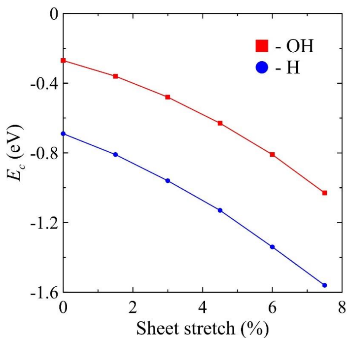
Рисунок 4. Зависимость энергии адсорбции E_c атома Н и группы ОН на растянутый графен от его деформации (предполагается одновременная деформация по обеим осям).
