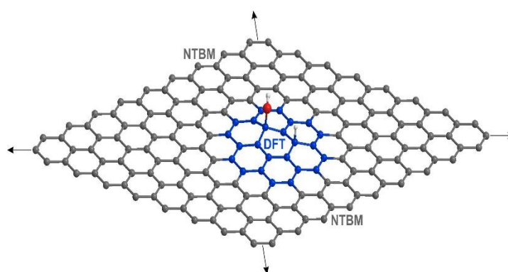
Рисунок 3. Схематичное изображение модели QM1/QM2, применяемой к напряженному графену. Область вблизи места адсорбции радикалов описывается в рамках теории функционала электронной плотности (DFT), а периферийная область – в рамках специально параметризованной неортогональной модели сильной связи (NTBM).
