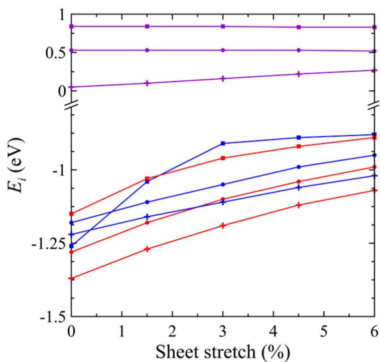
Рисунок 5. Энергии взаимодействия двух радикалов, одновременно адсорбированных на одном и том же углеродном шестиугольнике свободного и растянутого графенового листа в орто (красный), пара (синий) и мета (фиолетовый) положениях. Круги, квадраты и кресты соответствуют парам радикалов Н и Н; ОН и ОН; Н и ОН.
