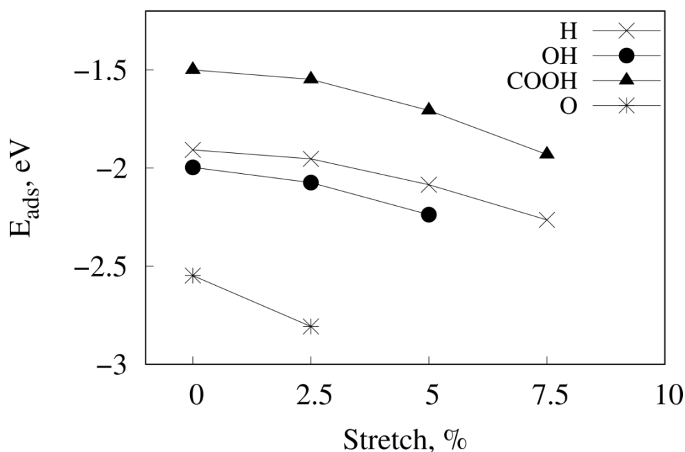
Рисунок 13. Зависимость энергии адсорбции радикалов H, OH, COOH и O от величины обратимого растяжения легированного азотом графена.
