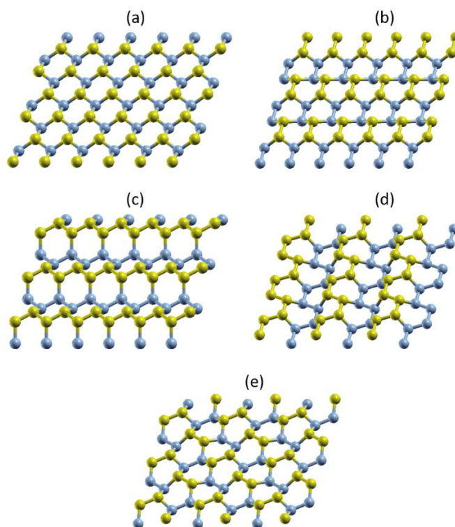
Рисунок 6. Пять возможных полиморфов А (a), В (b), С (c), D (d) и Е (e) полностью функционализированного графена с кристаллографически эквивалентными узлами. Желтые и синие круги представляют собой атомы углерода, связанные с радикалами, расположенными на верхней и нижней сторонах листа соответственно. Сами радикалы не показаны.
