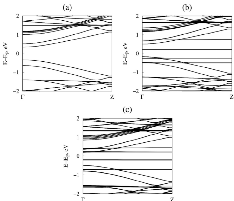
Рисунок 16. Зонные структуры для углеродной нанотрубки (14,0) (a) и пиподов на ее основе, содержащих фуллерены D_{6h}-C_{36} (b) и D_{2d}-C_{36} (c).
