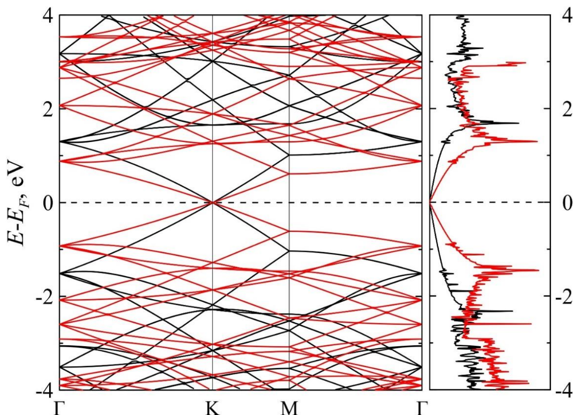
Рисунок 1. Графики зонной структуры (слева) и плотности состояний (справа) для ненапряженного графена (черная линия) и для графена, равномерно растянутого на 20% (красная линия). Буквами \Gamma , K и M обозначены характерные точки высокой симметрии в зоне Бриллюэна: \Gamma соответствует центру зоны Бриллюэна, K – точка Дирака.
