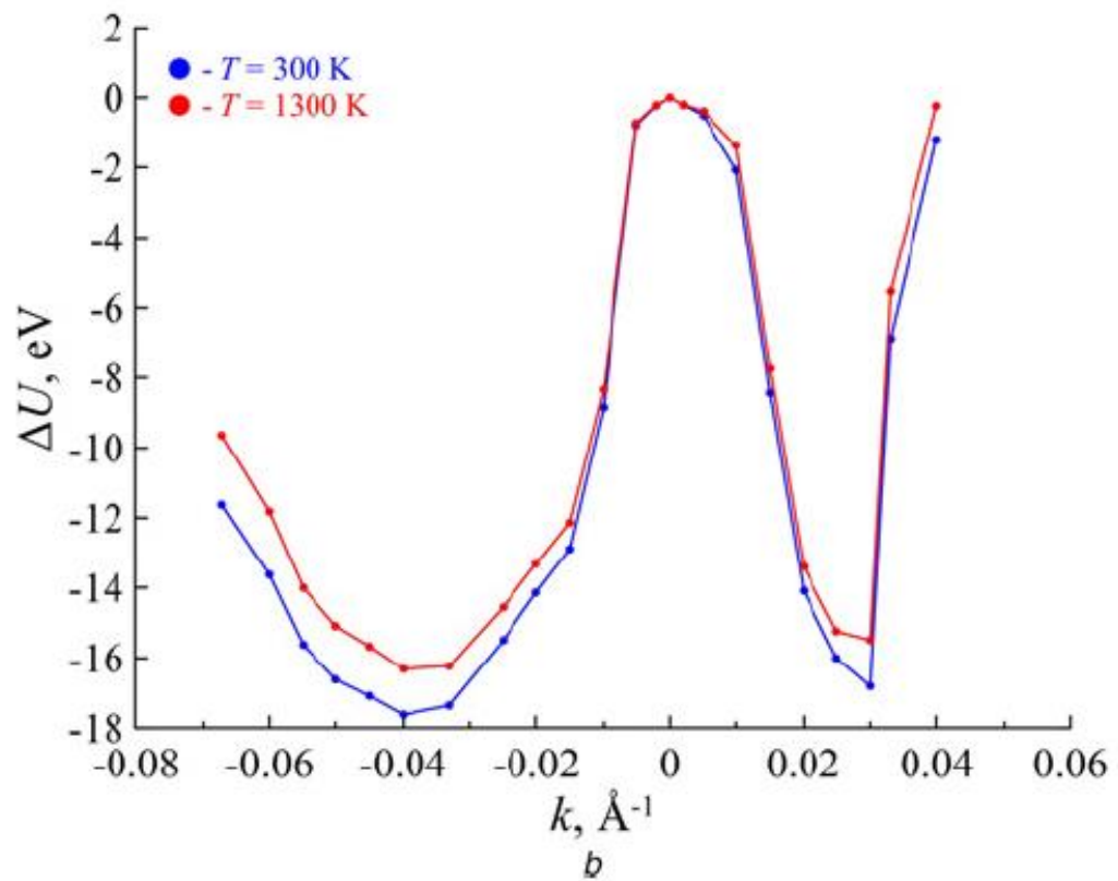
Рисунок 15. Средняя потенциальная энергия \Delta U изогнутого листа \text{C}_{678}\text{Ni}_{304} как функция его кривизны k в направлении зигзаг (a) или кресло (b) при температуре 300 K (синие кривые) и 1300 K (красные кривые). За точку отсчета энергии принимается энергия плоского листа.
