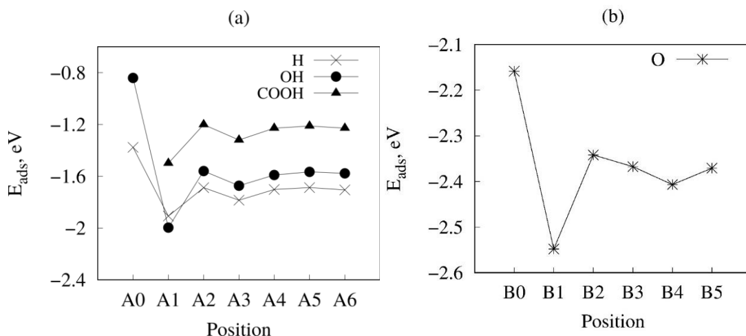
Рисунок 12. Энергии адсорбции E_{ads} радикалов H, OH, COOH (a) и O (b) для их различных взаимных расположений на поверхности N-легированного графена относительно замещающего атома азота.
