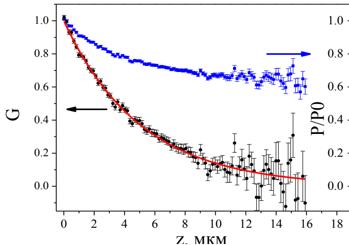
Рис.5 Изменение поляризации P/P_0 и СЭМУРН сигнал G в зависимости от спин-эхо длины z на ядрах HeLa. Данные аппроксимированы функцией P(z) = \exp(I\sigma(\exp(-z/\xi) - 1)) , \xi = (5.1 \pm 0.1) \cdot 10^3 \text{ nm} , \sigma I = 0.46 \pm 0.01 .
