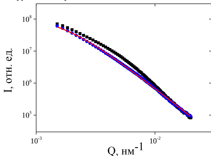
Рис.6 Ультра малоугловое рассеяние нейтронов на изолированных (синие точки) и агломерированных (черные точки) ядрах HeLa.
