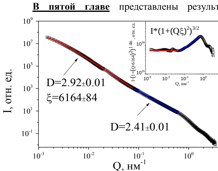
Рис.4 Малоугловое рассеяние нейтронов на ядрах HeLa. Интенсивность рассеяния нейтронов в диапазоне переданных импульсов 1.5 \cdot 10^{-3} \div 2 \cdot 10^{-2} \text{ nm}^{-1} — данные установки KWS-3, MLZ, Гархинг, Германия. Интенсивность рассеяния нейтронов в диапазоне переданных импульсов 2 \cdot 10^{-2} \div 3 \cdot 10^0 \text{ nm}^{-1} — данные установки D11, ILL, Гренобль, Франция.
