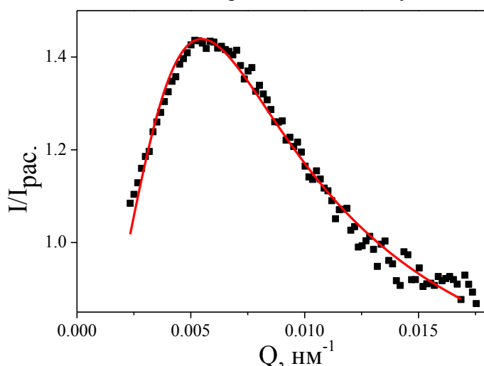
Рис.7 Отношение интенсивности рассеяния на агломерированных ядрах HeLa к интенсивности рассеяния на изолированных ядрах HeLa.
