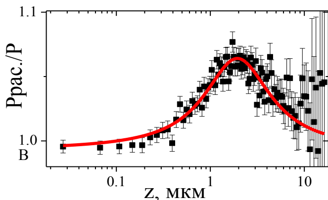
Рис.8 Отношение рассчитанной поляризации на изолированных ядрах HeLa к экспериментальной поляризации для агломерированных ядер HeLa.
