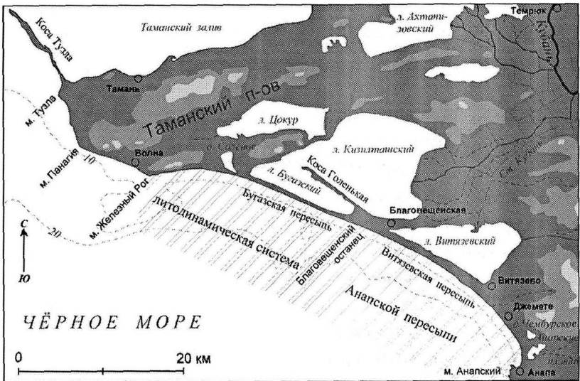
Рис. 1. Схема района литодинамической системы Анапской пересыпи
