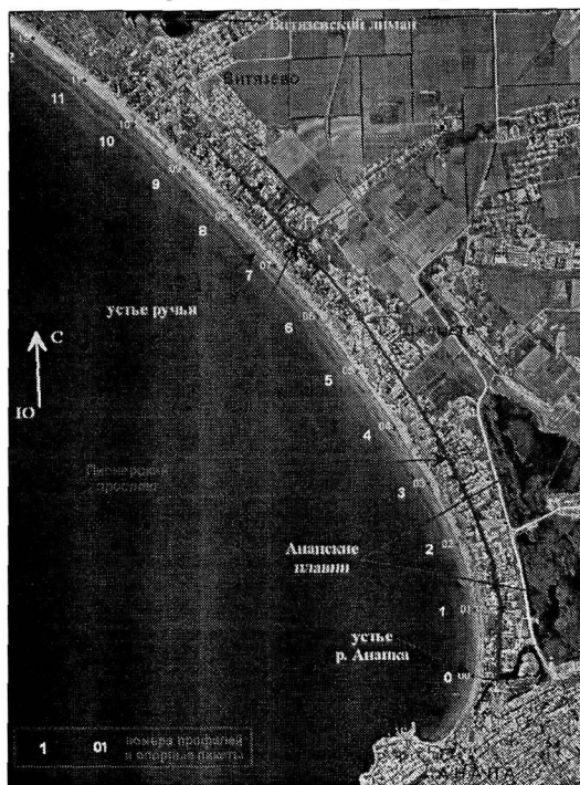
Рис. 2 – Схема организации полевых работ (0-11 – номера профилей)
