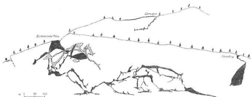
Рис. 2. Разрез Долганской карстовой системы (По А.В. Осинцеву с дополнениями А.Д. Ботвинкина и О.Н. Морозова)
