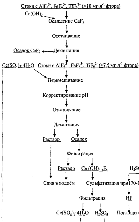
Рисунок 3 – Принципиальная технологическая схема очистки сточных вод от примеси фтора, присутствующего в виде комплексов с титаном, железом, алюминием, до норм, установленных для водоёмов питьевого назначения
