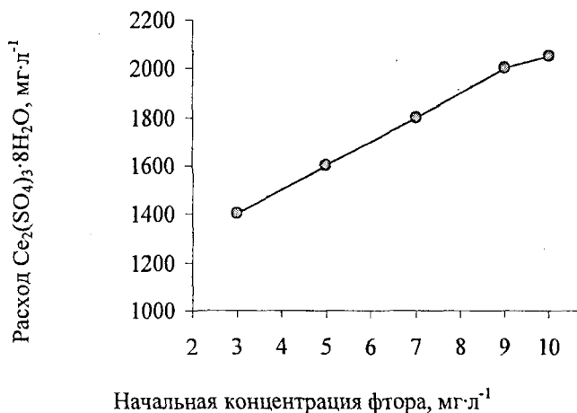
Рисунок 1 – Минимальный расход \text{Ce}_2(\text{SO}_4)_3 \cdot 8\text{H}_2\text{O} , обеспечивающий очистку стоков до остаточного содержания фтора 0.75 \text{ мг}\cdot\text{л}^{-1} (фтор в виде \text{AlF}_6^{3-} )
