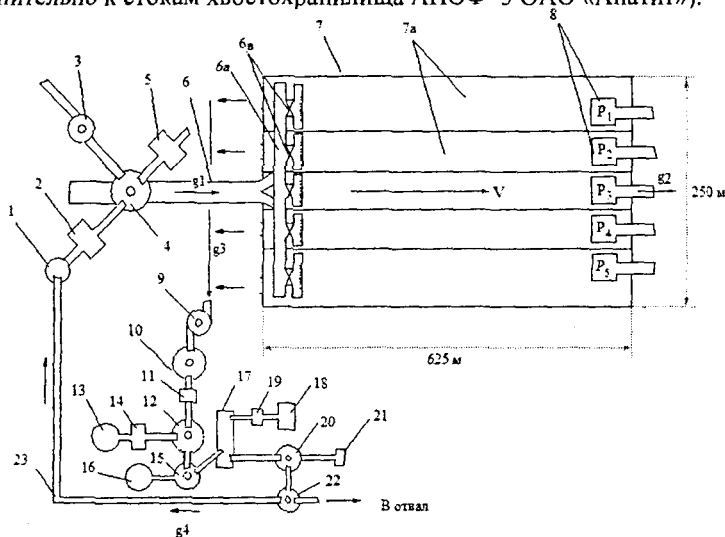
Рисунок 4 – Принципиальная схема цепи аппаратов комплекса для очистки стоков:
