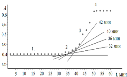
Рисунок 3 – Зависимость A_{350}=f(t) для раствора (CF_3COO)_2Cd \cdot nH_2O –ТAA–ЭА, C_{Cd}=2,00 \cdot 10^{-3} моль/л, мольное соотношение Cd:ТAA=1:4, l = 1,00 см
