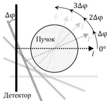
Рисунок 1 – Схема регистрации энергетического распределения ионизирующего излучения в поперечном сечении пучка методом многоуглового сканирования
