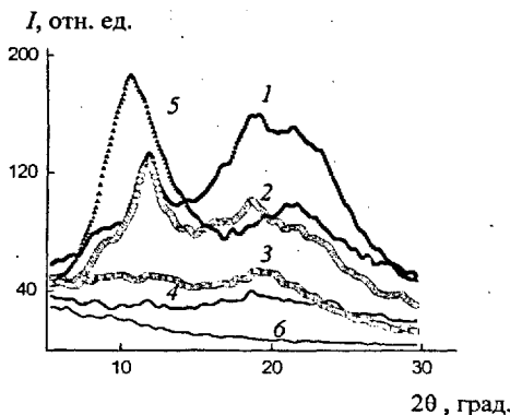
Рис. 8. Рентгеновские дифрактограммы пленок хитозана, полученных из водно-уксусно-кислых растворов: 1 – хитозан, (рН пленкообразующего раствора 3.8); 2 – смесь гомополимеров [хитозан]:[ПВП] = 1.0:0.25 осново-моль (рН пленкообразующего раствора 3.8); 3, 4 – привитый сополимер ХТЗ-ВП (1:1 и 0.25:1 осново-моль соответственно); 5 – ПВП; 6 – кювета без пленки.
