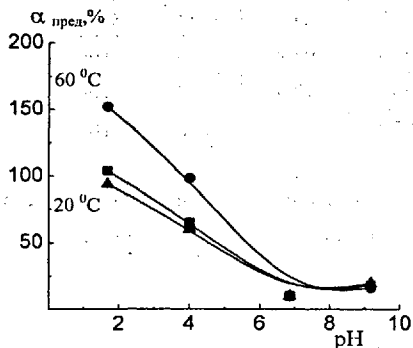
Рис. 10. Зависимость предельной степени набухания ( \alpha_{\text{пред}} ) геля на основе ХТЗ, сшитого ДАТФ, от pH среды (буферный раствор) при различных температурах. [\text{ДАТФ}]/[\text{ХТЗ}] = 0,05 ; [\text{ДО}] = 1,68 \times 10^{-3} \text{ M} ; [\text{УК}] = 0,225 \text{ M} .
