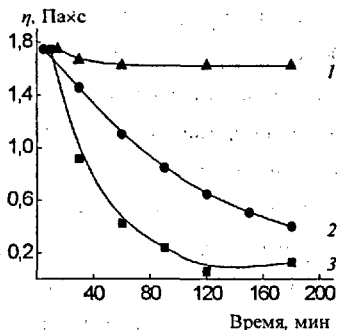
Рис. 1. Изменение вязкости растворов хитозана ( [\text{ХТЗ}]=0.186 моль/л) от времени в присутствии различных концентраций [(\text{NH}_4)_2\text{S}_2\text{O}_8] : 1 - 1 \times 10^{-4} , 2 - 1.4 \times 10^{-3} , 3 - 1 \times 10^{-2} моль/л, pH = 4.2, 293 К (здесь и далее [\text{ХТЗ}] - концентрация звеньев в цепях хитозана).
