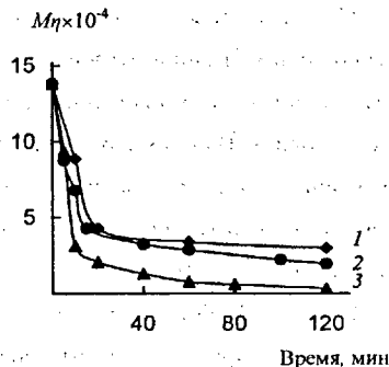
Рис. 2. Изменение средневязкостной молекулярной массы хитозана ( [\text{ХТЗ}]=0.186 моль/л) в присутствии инициатора ( [(\text{NH}_4)_2\text{S}_2\text{O}_8] = 1.3 \times 10^{-2} моль/л) от времени в зависимости от температуры: 1 - 323 К, 2 - 333 К, 3 - 353 К.
