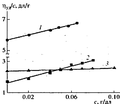
Рис. 6. Зависимость приведенной вязкости от концентрации полимера: 1 - исходный хитозан, 2 - хитозан после ультразвуковой деструкции в течение 15 мин, 3 - продукт реакции.
