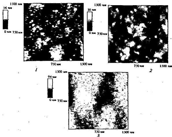
Рис. 9. Топография поверхности пленки хитозана (1), смеси гомополимеров ХТЗ и ПВП = 1:1 осново-моль (2), привитого сополимера ХТЗ-ВП (1:1 осново-моль) (3).
