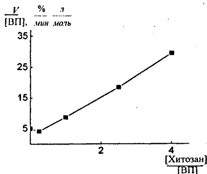
Рис. 4. Зависимость приведенной скорости превращения ВП от отношения начальных концентраций хитозана и ВП. [Хитозан] = 0.12 осново-моль/л, [\text{CH}_3\text{COOH}] = 0.3 моль/л, [(\text{NH}_4)_2\text{S}_2\text{O}_8] = 4 \times 10^{-3} моль/л, 333 К.
