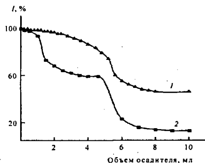
Рис. 7. Зависимость процента светопропускания растворов осажденного продукта полимеризации АА в присутствии хитозана (1) и смеси хитозан- ПАА (1:1)(2) от объема добавленного осадителя - ацетона. Концентрация полимера 0.5 мас.%, 293 К.
