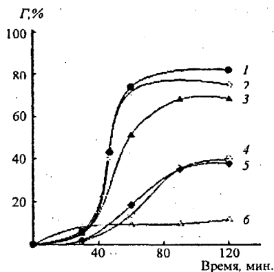
Рис. 3. Зависимость глубины превращения АА в растворах хитозана от времени при различном значении pH реакционной среды (pH=5.5 (1,6), pH=4.2 (2-5)) и различном мольном отношении АА и звеньев хитозана: 1 - [\text{AA}]:[\text{ХТЗ}] = 3 ; 2 - [\text{AA}]:[\text{ХТЗ}] = 3 ; 3 - [\text{AA}]:[\text{ХТЗ}] = 2 ; 4 - [\text{AA}]:[\text{ХТЗ}] = 0.33 ; 5 - [\text{AA}]:[\text{ХТЗ}] = 1 ; 6 - [\text{AA}] = 0.56 моль/л (в отсутствие \text{ХТЗ} ); [\text{ХТЗ}] = 0.186 ; [\text{CH}_3\text{COOH}] = 0.25 ; [(\text{NH}_4)_2\text{S}_2\text{O}_8] = 1.4 \times 10^{-3} моль/л, 323 К.
