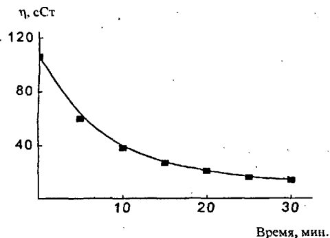
Рис. 5. Изменение вязкости в процессе ультразвуковой деструкции 3%-го раствора хитозана в присутствии 0.01 мас.% гидрохинона, 273-275 К.
