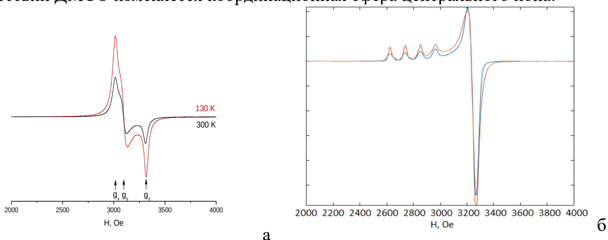
Рис. 5. ЭПР спектр \text{Cu}(\text{HL}^3)_2 : а – поликристаллический образец при 130 (красная линия; \nu=9.4722 Гц) и 300 К (черная линия, \nu=9.4708 Гц); спектры описаны модельными спектрами для S=1/2 , g\{2.245, 2.186, 2.043\} , б – растворы в ДМСО при 130 К, 9.472194 Гц (красная линия) и модельный спектр для S=1/2 , g\{2.085, 2.085, 2.42\} , A\{0.001, 0.001, 0.0125\}\text{см}^{-1} .
