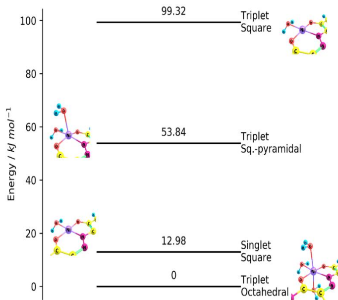
Рис. 6. Относительные энергии комплексов \text{Ni}(\text{II}) с \text{H}_2\text{L}^3 в различных окружениях и мультиплетных состояниях (DFT расчеты)
