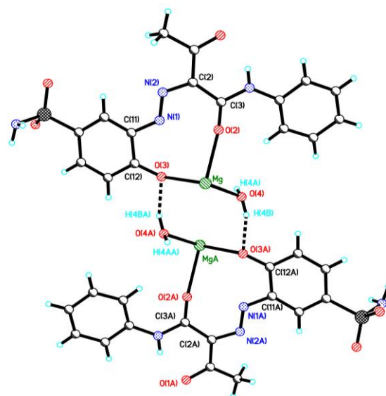
Рис. 3. Координационное окружение атома Mg(II) (а) и формирование центросимметричного димера в структуре Mg(L^3) \cdot H_2O (б).
