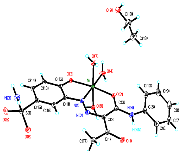
Рис 4. Молекулярная структура [Ni(L 3 )·(H 2 O) 3 ]·C 2 H 5 OH.
