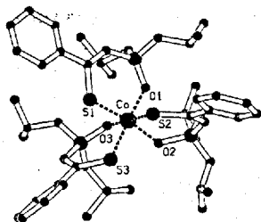
Рисунок 6. Молекулярная структура комплекса 10v .
