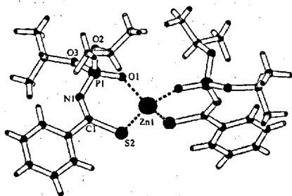
Рисунок 2. Молекулярная структура комплекса 10г .
