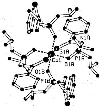
Рисунок 3. Молекулярная структура комплекса 10б .
