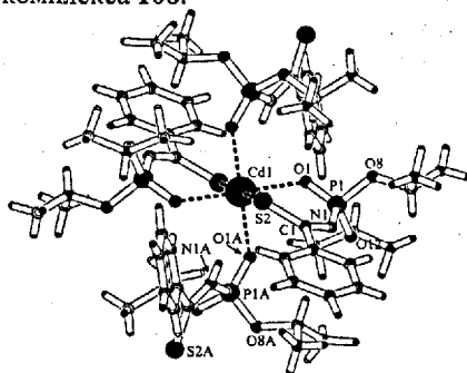
Рисунок 5. Молекулярная структура комплекса 10е .
