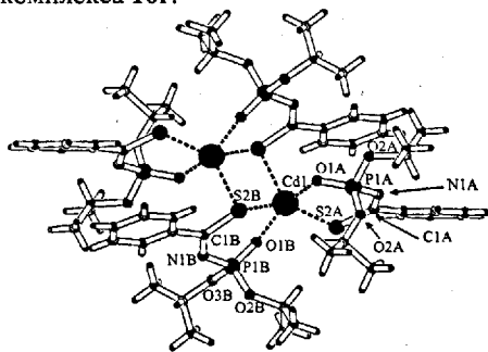
Рисунок 4. Молекулярная структура комплекса 10д .
