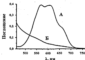
Рисунок 7. УФ спектр видимой области комплексов 10а (кривая А) и 11ж (кривая Б).
