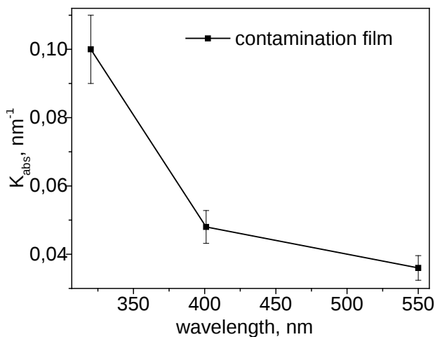
Рис. 2. Коэффициент поглощения контаминационной плёнки, формирующейся под электронным пучком в процессе облучения образцов YAG.
