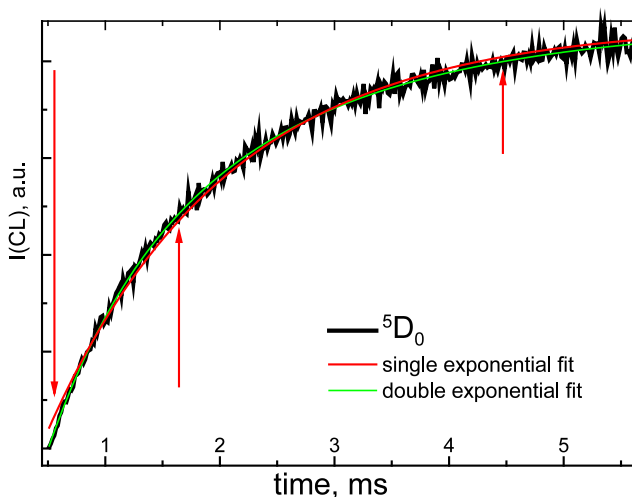
Рис. 5. Кинетика разгорания уровня ^5D_0 Eu 3+ в монокристалле и нанокерамике на основе YAG.
