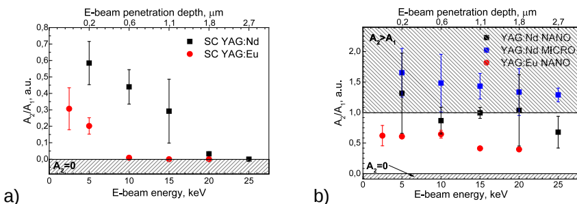
Рис. 4. Зависимость отношения вклада короткого времени затухания к длинному ( A_2/A_1 ) от энергии электронного пучка в образцах а) монокристаллов; б) керамики.
