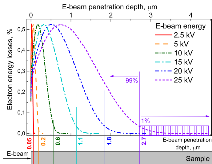
Рис. 1. Распределение потерь энергии электронов по глубине проникновения электронного пучка при различных энергиях в YAG. Цифры у нижней оси указывают глубину проникновения электронного пучка, при которой теряется 99% энергии электронов.
