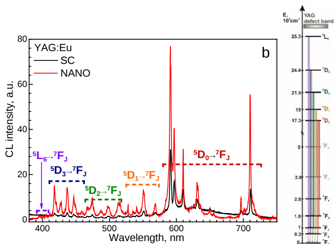
Рис. 3. КЛ спектры образцов (слева) а) YAG:Nd и б) YAG:Eu и их интерпретация согласно схемам энергетических уровней РЗИ (справа).
