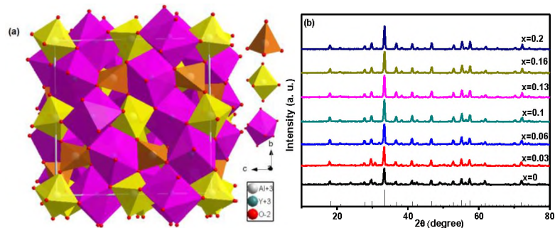
Рисунок 2 – Структура (а) и рентгенограммы люминофоров \text{YAG:0.1Ce}^{3+} , x\text{Mn}^{2+} , x\text{Si}^{4+} ( x = 0-0.2 мол.%) с различным содержанием пары \text{Mn}^{2+} - \text{Si}^{4+} (б).
