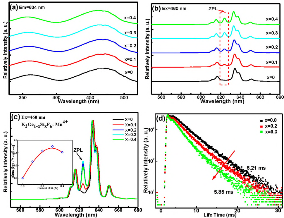
Рисунок 13. Спектры ВФЛ (мониторинг при \lambda_{em} = 634 nm) при комнатной температуре (а), спектры ФЛ, возбуждаемые при \lambda_{ex} = 460 nm (б), нормированные спектры излучения (на вставке - соотношение интенсивности ZPL/ \nu_6 (634 nm) (с), кинетики затухания люминесценции \text{Mn}^{4+} при комнатной температуре в KGSFM при x = 0, 0.2, 0.3 (д).
