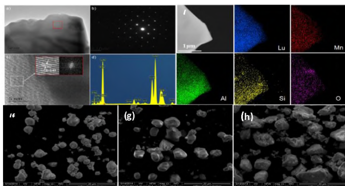
Рисунок 6 – ПЭМ-изображение (а), SAED-изображение (б), ПЭМБВР-изображение (с) и обнаруженная картина EDS (д) в ЛюАГ: \text{Ce}^{3+} , \text{Mn}^{2+} , \text{Si}^{4+} ; ПЭМ-изображение и EDS элементное картирование частицы ЛюАГ: \text{Ce}^{3+} , \text{Mn}^{2+} , \text{Si}^{4+} (е); СЭМ-изображения морфологии люминофоров ЛюАГ: \text{Ce}^{3+} , x\text{Mn}^{2+} , \text{Si}^{4+} : x = 0 мол.% (ф), x = 0,1 мол.% (г), x = 0,2 мол.% (h)
