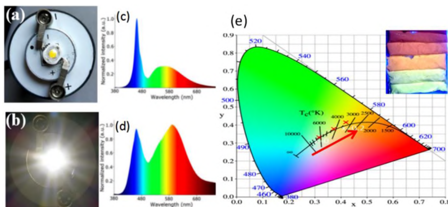
Рис. 4 - Фото СД в нерабочем (b) и рабочем (a) состояниях, спектры излучения СД с люминофорами из смеси ИАГ:Ce 3+ и ИАГ:Ce 3+ , Mn 2+ , Si 4+ (x = 0.2 моль%) и их коррелированные цветовые температуры на диаграмме МКО (e) (на вставке – фото излучения люминофоров).
