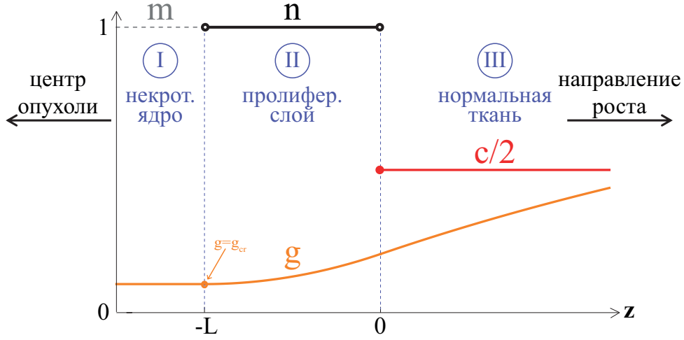
Рис. 2 — Форма решения уравнений (1), которое ищется аналитически.
