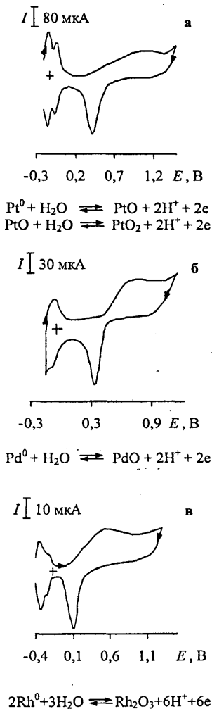
Рис. 1. Циклические вольтамперограммы, полученные на Pt-CU (а), Pd-CU (б) и Rh-CU (в) на фоне 0.1 М раствора H_2SO_4
