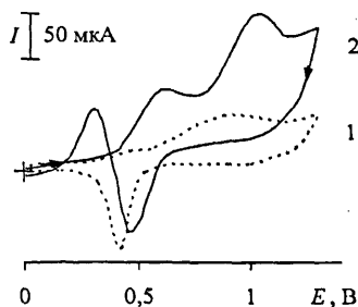
Рис. 12. Циклические вольтамперограммы, полученные на Pt-CU в отсутствие (1) и присутствии (2) этанола ( C = 5 \times 10^{-2} М) (2) на фоне 0.1 М H_2SO_4
