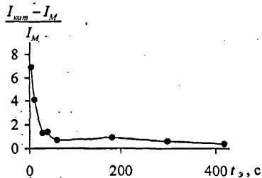
Рис. 11. Зависимость каталитического эффекта при окислении 5 \times 10^{-3} М щавелевой кислоты на электроде Pd-CU от времени электролиза на фоне 0.1 М раствора \text{H}_2\text{SO}_4
