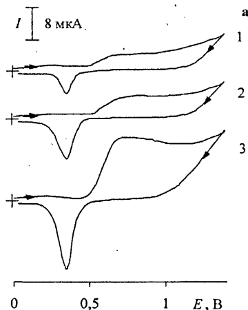
Рис. 3. Циклические вольтамперограммы (а) и АСМ изображения поверхности (б, в) УПЭ с электроосажденным палладием в течение 15 (1а, б), 30 (2а), 60 (3а, в) с из 5 \times 10^{-3} М раствора \text{PdCl}_2 на фоне 0.1 М раствора \text{H}_2\text{SO}_4
