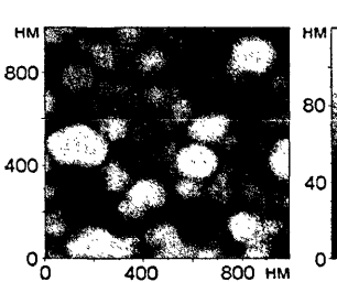
Рис. 3. Циклические вольтамперограммы (а) и АСМ изображения поверхности (б, в) УПЭ с электроосажденным палладием в течение 15 (1а, б), 30 (2а), 60 (3а, в) с из 5 \times 10^{-3} М раствора \text{PdCl}_2 на фоне 0.1 М раствора \text{H}_2\text{SO}_4
