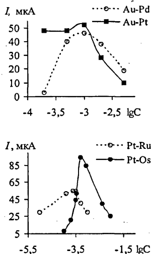
Рис. 16. Зависимость тока пика окисления биметаллического композита от концентрации одного из компонентов бинарной системы
