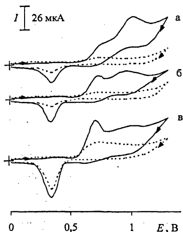
Рис. 10. Циклические вольтамперограммы окисления 5 \times 10^{-3} М щавелевой кислоты, полученные на СУ с электроосажденным палладием в течение 15 (а), 30 (б), 60 (в) с на фоне 0.1 М раствора \text{H}_2\text{SO}_4
