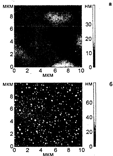
Рис. 8. АСМ изображения поверхности электродов НФ-ВОИПГ (а) и Pd-НФ-ВОИПГ (б); палладий электроосадили из раствора 1 \times 10^{-4} М PdCl 2 в течение 10 с
