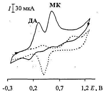
Рис. 19. Циклическая вольтамперограмма, полученная на Au-Os-Cu в растворе, содержащем ДА и МК ( C = 5 \times 10^{-3} М) на фоне фосфатного буфера pH 6.9, пунктирная линия – фоновая кривая
