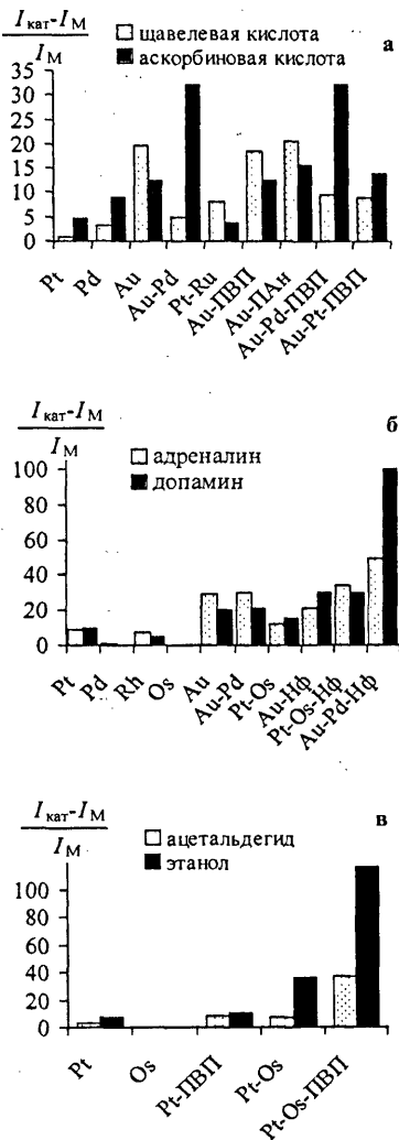
Рис. 17. Зависимость каталитического эффекта от природы медиаторной системы для аскорбиновой и шавелевой кислот (а), допамина и адреналина (б), этанола и ацетальдегида (в); фон 0.1 M H 2 SO 4
