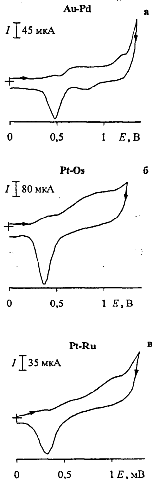
Рис. 14. Циклические вольтамперограммы окисления осадков, полученных из бинарных систем Au-Pd (а), Pt-Os (б) и Pt-Ru (в) на фоне 0.1 M H 2 SO 4
