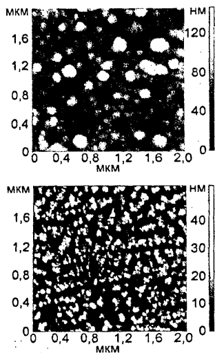
Рис. 5. АСМ изображения поверхности ВОПГ с электроосажденным в течение 5 с палладием из раствора 5 \times 10^{-3} М (а) и 1 \times 10^{-4} М (б) \text{PdCl}_2
