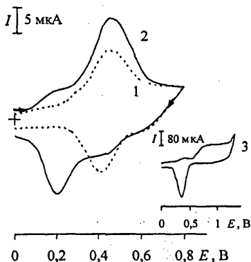
Рис. 9. Циклические вольтамперограммы, полученные на ПАН-СУ (1) и Pd-ПАН-СУ (2,3) на фоне 0.1 М \text{H}_2\text{SO}_4 ; палладий электроосаждали из 5 \times 10^{-3} М раствора \text{PdCl}_2 в течение 5 (2), 180 (3) с
