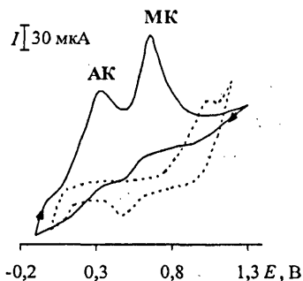
Рис. 18. Циклическая вольтамперограмма, полученная на Au-Ru-Cu в растворе, содержащем АК и МК ( C = 5 \times 10^{-3} М) на фоне фосфатного буфера pH 6.9, пунктирная линия – фоновая кривая
