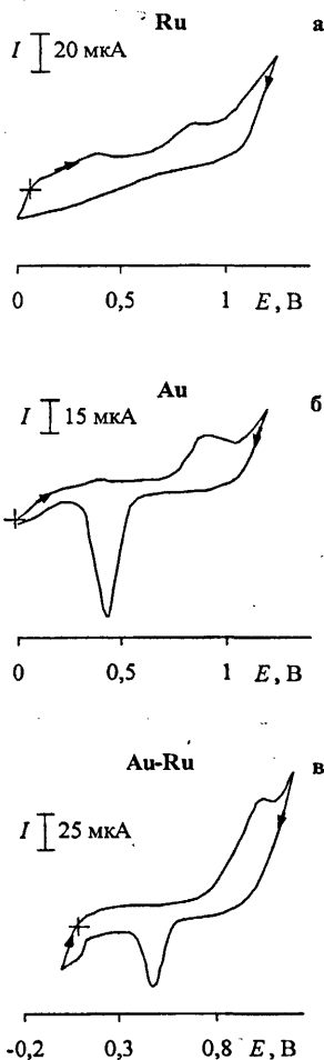
Рис. 15. Циклические вольтамперограммы, полученные на электродах Ru-CU (а), Au-CU (б) и Au-Ru-CU (в) на фоне фосфатного буферного раствора с pH 6.9
