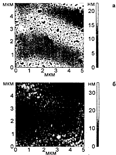
Рис. 7. АСМ изображения поверхности электродов ПВП-ВОИПГ (а) и Pd-ПВП-ВОИПГ (б); палладий электроосадили из раствора 1 \times 10^{-4} М PdCl 2 в течение 10 с
