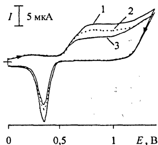
Рис. 6. Циклические вольтамперограммы, полученные на электродах Pd-ПВП-ВОПГ (1), Pd-ВОПГ (2), Pd-НФ-ВОПГ (3) в 0,1 М растворе \text{H}_2\text{SO}_4
