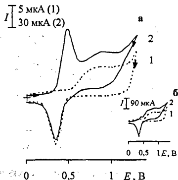
Рис. 13. Циклические вольтамперограммы, полученные на Pd-CU в отсутствие (1) и присутствии (2) допамина ( C = 5 \times 10^{-3} M) на фоне 0.1 M H_2SO_4 ; палладий электроосадили в течение 5 (а), 180 (б) с
