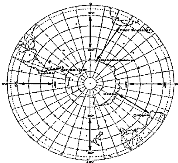
Рис.6 Расположение станций и сечений по которым определялись разности давлений.
