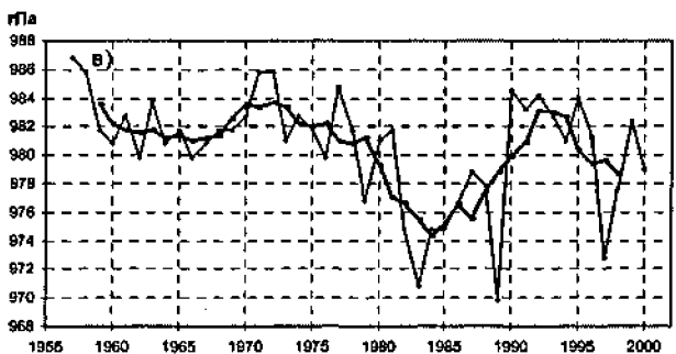
Рис.2 Изменения давления за зимний период в циклонических центрах действия атмосферы Южного полушария: Южно-Антарктический (а), Индоокеанский (б), Южно-Тихоокеанский (в). Жирной линией показаны их 5-летние скользящие средние.
