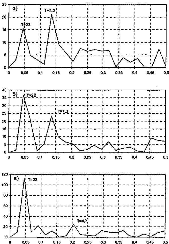
Рис.3 Спектры многолетней изменчивости давления в центрах действия атмосферы Южного полушария: Южно-Атлантический (а), Индоокеанский (б), Южно-Тихоокеанский (в).
