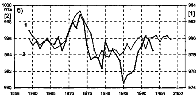
Рис.5 Сопоставления 5-летних скользящих средних значений давления за зимний период в центре Алеутской депрессии (1) с изменениями давления (2) в Южно-Тихоокеанской депрессии (а) и Индоокеанской (б).
