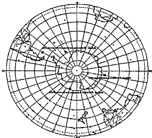
Рис. 1 Среднегодовое положение циклонических центров действия атмосферы в Южном полушарии.
