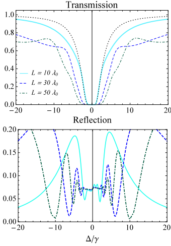
Рис. 1 — а) Зависимость коэффициентов прохождения и отражения от отстройки пробного излучения \Delta = \omega - \omega_0 для неоднородного распределения плотности атомов в конденсате, где \omega_0 — резонансная частота атомного перехода. Пунктиром изображена реперная зависимость для коэффициента прохождения света через оптически плотный слой невырожденного газа той же плотности, что и рассматриваемый конденсат. б) Зависимость коэффициента отражения, описываемого тем же параметром порядка, в точке резонанса \omega = \omega_0 , как функция 2\pi/\Delta q (в единицах резонансной длины волны \lambda_0 ) для образцов различных длина L .
