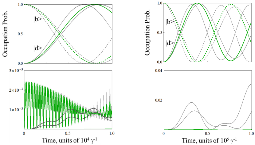
Рис. 2 — а) Верхний график : Временная зависимости вероятностей заселения базового состояния |b\rangle (пунктирные кривые) и конечного состояния |d\rangle (сплошные кривые), приведенные для отстройки от оптического резонанса \Delta = -1000\gamma . Нижний график : Несовершенство переселения и утечка из основного канала рассеяния, пояснения см. текст. б) Те же зависимости для отстройки \Delta = -5000\gamma .
