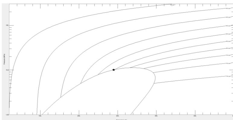
Рисунок 5 – Р-Т диаграмма газоконденсатной смеси Ковыктинского ГКМ в соотношении 9:1
