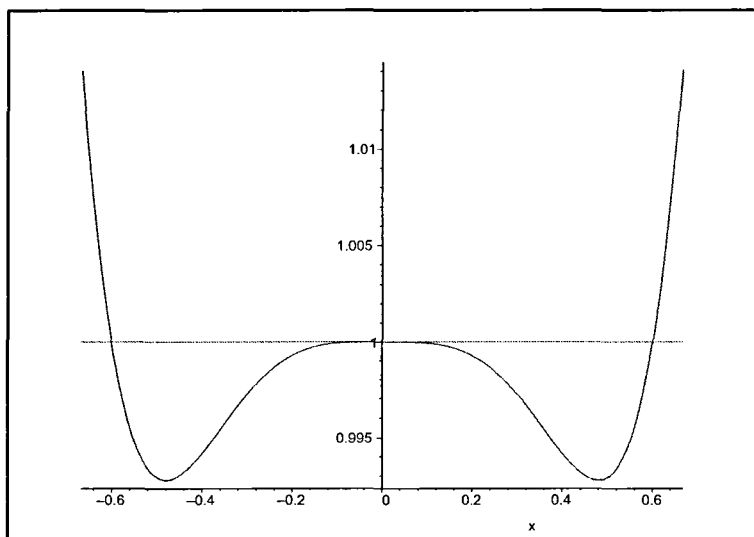
Рис. 4: График \varphi(x) . Случай (4, 6). Интервал \left[-\frac{2}{3}, \frac{2}{3}\right]
