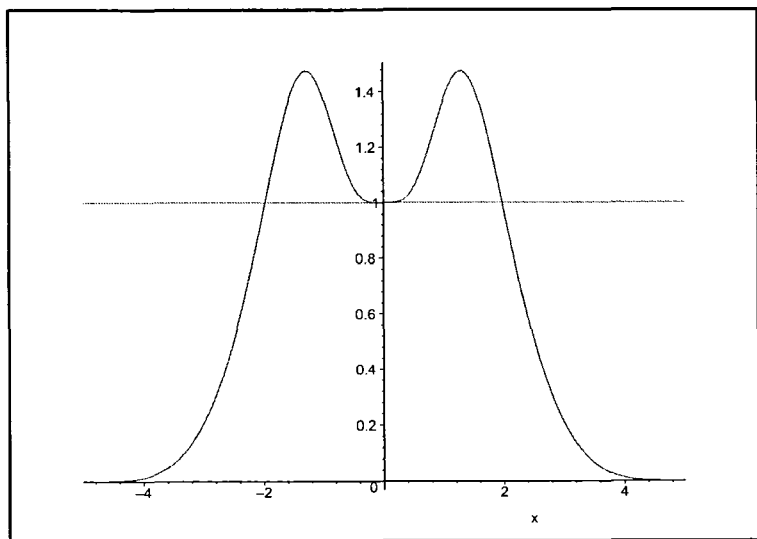
Рис. 2: График функции \varphi(x) . Случай (3, 5)
