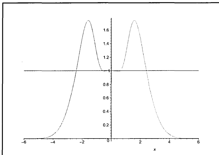
Рис. 3: График функции \varphi(x) . Случай (4, 6)
