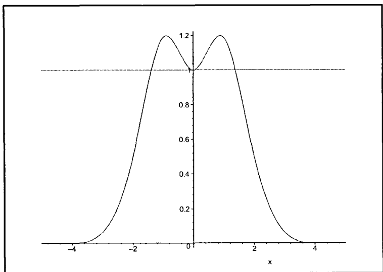
Рис. 1: График функции \varphi(x) . Случай (2, 4)
