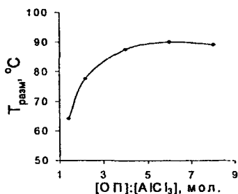
Рис.3 Зависимость T_{\text{разм}} НПС от мольного соотношения ОП:AlCl 3 . T_{\text{дезакт}}=75^{\circ}\text{C} .
