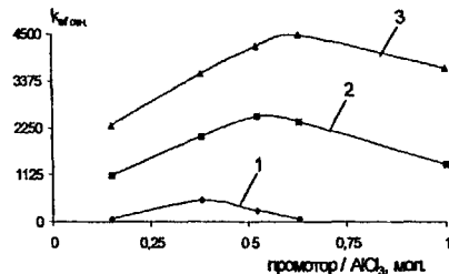
Рис.1 Влияние промотирующей добавки {вода (1) и смесь вода:ацетон (2, 3)} на СП_{отн} (а) и k_{ef\ отн} (б). [H_2O]:[AlCl_3] , мол.: 0,25 (2), 0,14 (3).
