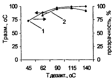
Рис.4 Зависимость прозрачности (1) и T_{\text{разм}} (2) НПС от T_{\text{дезакт.}} ОП:AlCl 3 =5:1, мол.
