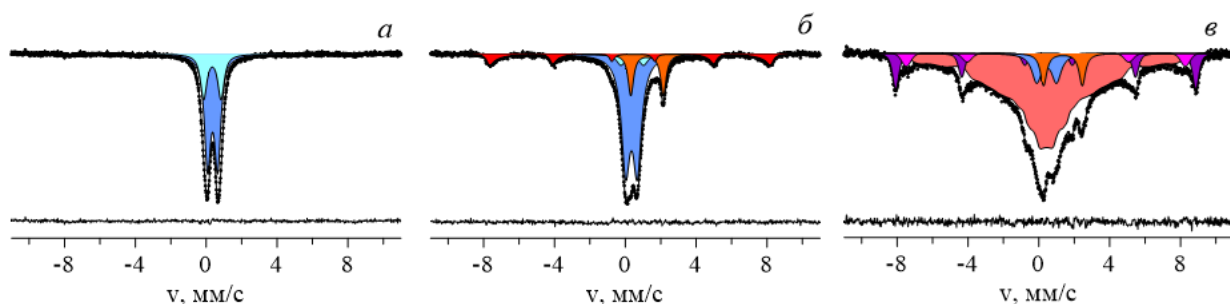
Рисунок 1. Мессбауэровские спектры ядер ^{57}\text{Fe} в структуре минералов а) контрольного образца ферригидрита ( T = 295 К), образца, полученного в результате роста бактерии F. ferrireducens , б) ( T = 295 К), в) ( T = 82 К).
