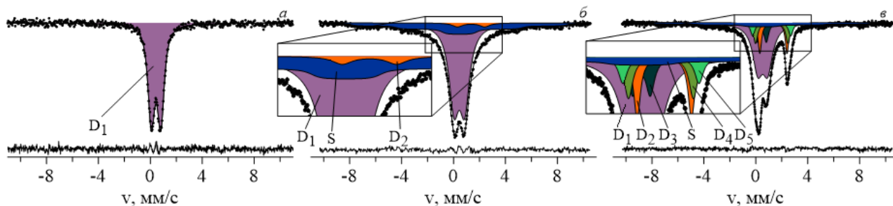
Рисунок 2. Мессбауэровские спектры, измеренные при температуре T = 82 \text{ K} : (a) контрольного абиогенного образца ферригидрита; опытных образцов, полученных на (б) 5-й день; (в) 34-й день инкубации синтрофной культуры на ферригидрите.
