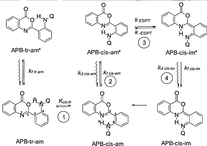
Рисунок 2. Схема процессов в основном и возбужденном состояниях аминифенилбензоксазионов.
