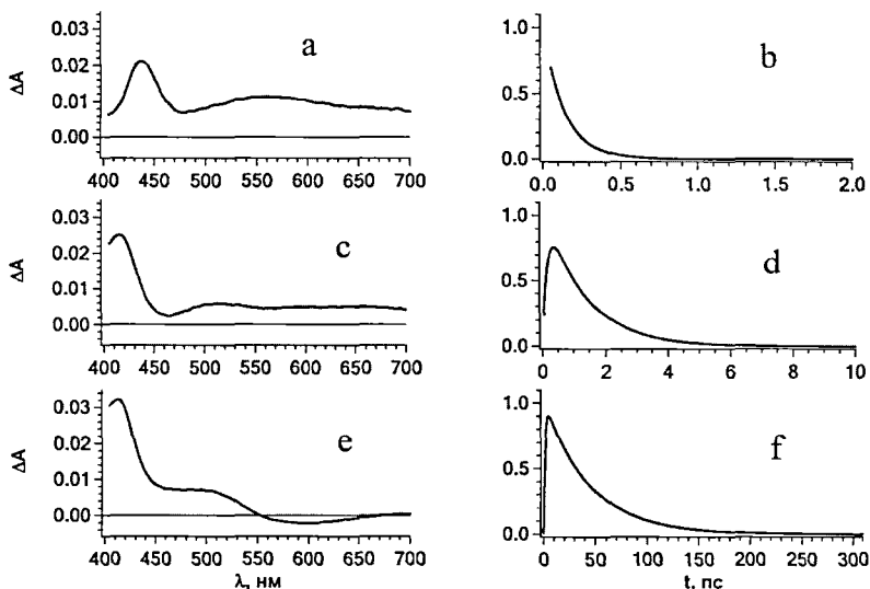
Рисунок 5. Спектры и кинетические кривые превращения интермедиатов для соединения APB2: APB2-am^* – a, b; APB2-am_r^* – c, d; APB2-im^* – e, f.
