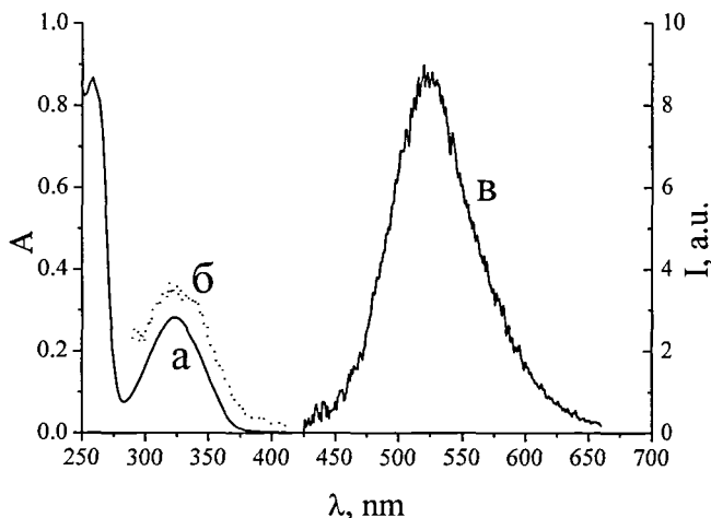
Рисунок 6. Спектры поглощения (а), возбуждения (б) и испускания (в) флуоресценции ТАЛ в этаноле (для нейтрализации анионной формы раствор подкисляли C(H_2SO_4)=10^{-3} моль/л).
