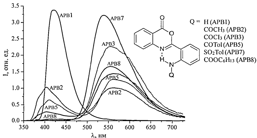
Рисунок 1. Спектры флуоресценции аминофенилбензоксазинов в метилциклогексане при комнатной температуре.
