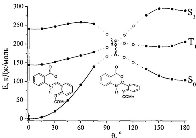
Рисунок 4. Зависимость потенциальной энергии продукта ВФПП APB2 от двугранного угла ( \theta ) между бензоксазиновым и замещенным фенильным фрагментами в S_0 , S_1 и T_1 состояниях (TDDFT).
