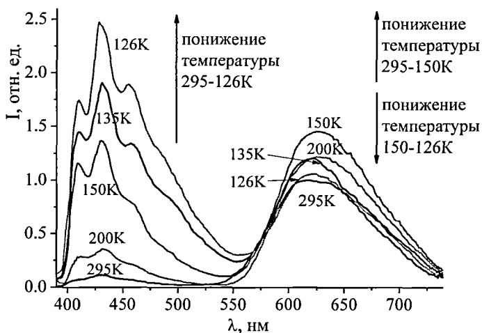
Рисунок 8. Спектры флуоресценции АВТН + в этаноле при разных температурах.
