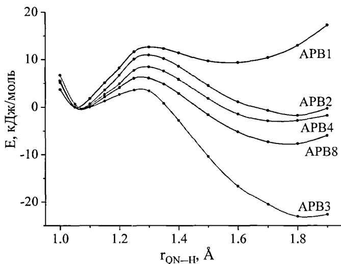
Рисунок 3. Зависимость потенциальной энергии аминифенилбензоксазинов от длины связи QN-H в возбужденном состоянии (х-МСQDPT2).
