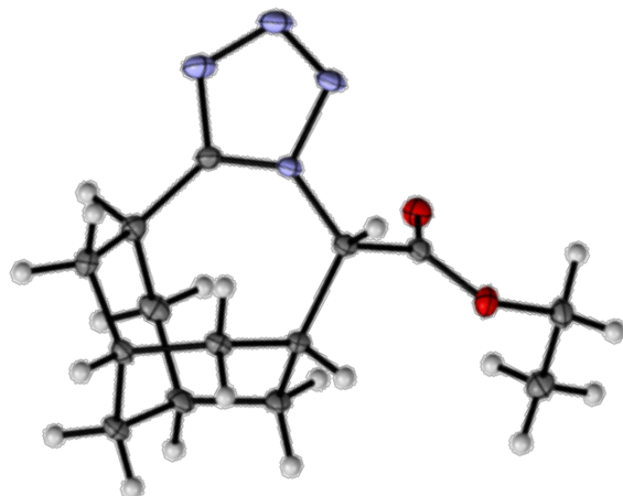
Рисунок 3. ORTEP-молекулярная структура тетразола 2.41 1 (CCDC 1552406) 2 в представлении эллипсоидами термических колебаний атомов с вероятностью
