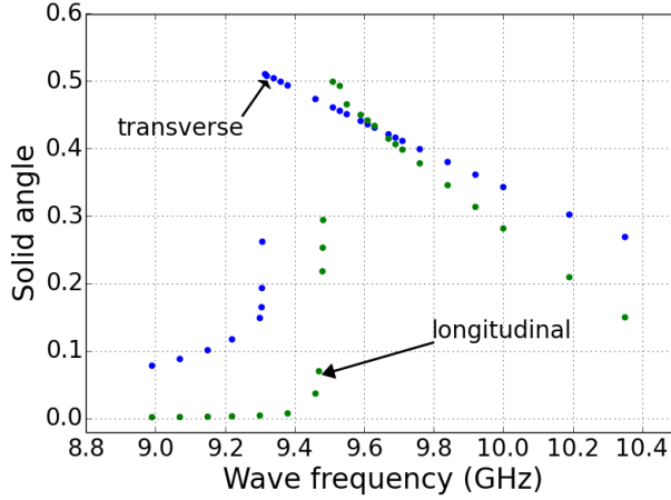
Рис. 1: Частотные зависимости телесного угла прецессии намагниченности в установившемся режиме в пучностях поперечных (transverse) и продольных (longitudinal) стоячих волн в плёнке \text{Fe}_{81}\text{Ga}_{19} .
