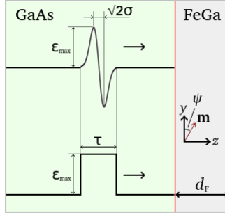
Рис. 6: Схематическое изображение биполярного и прямоугольного импульсов, используемых при моделировании гетероструктуры GaAs/Fe 81 Ga 19 . Время \tau обозначает длительность импульса, \varepsilon_{\max} – максимальную амплитуду деформаций в импульсе, а d_F – толщину плёнки Fe 81 Ga 19 .
