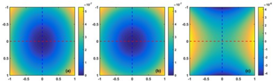
Рис. 2. Характерное поперечное распределение оптического пути \psi_{\Sigma}/k (м) (a), \psi_{noangledep}/k (м) (b), \psi_{astigm}/k (м) (c) в поперечном сечении ОЭ изготовленном из кристалла \text{CaF}_2 при \delta_c = 0 , \Phi = 0 в ориентации кристаллографических осей [001]. F_1 и F_2 – фокусы, для направлений по полярному углу \varphi = 0, \pi/2 , определяющие (\psi_{\Sigma})_{max} и (\psi_{\Sigma})_{min} .
