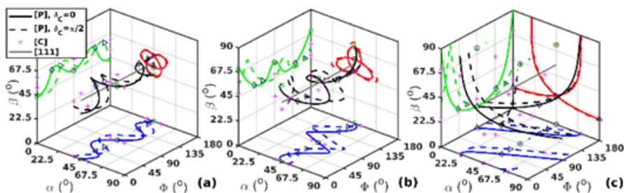
Рис. 3 Зависимости углов Эйлера ( \alpha , \beta , \Phi ) от параметра оптической анизотропии \xi = -0.2 (a), -0.8 (b), -4 (c) в случае \delta_c = 0 (проходной ОЭ или АЭ) и \delta_c = \pi/2 (МОЭ) для ориентации кристаллографических осей [P] и их проекции на плоскости ( \alpha , \beta ), ( \alpha , \Phi ) и ( \beta , \Phi ); направления кристаллографических осей [C] и [111]; точками показаны аналитически найденные решения [P].
