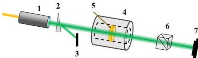
Рис. 8. Схема эксперимента по измерению постоянной Верде. 1 –лазеры с длинами волн 405, 532, 674, 808, 980 и 1064 нм, а также He-Ne-лазер с длиной волны 632.8 нм, 2 – шпатовый клин, 3 – поглотитель излучения, 4 – магнитная система, 5 – исследуемый образец, 6 – призма Глана, 7 – CCD-камера.
