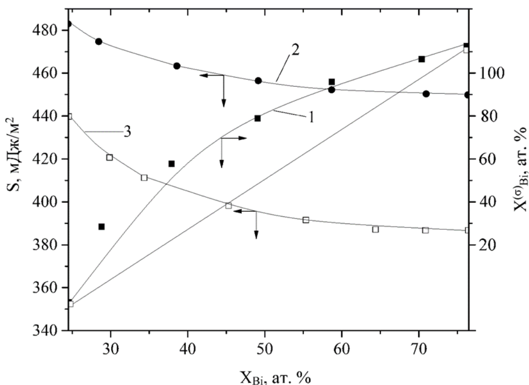
Рисунок 9 - Поверхностная сегрегация ( T = 623 K) в расплавах Tl-Bi, рассчитанная с учетом матричных эффектов (кривая 1) ( x_{Bi} , x^{(\sigma)}_{Bi} – объемная и поверхностная концентрация Bi). Поверхностное натяжение (623 K) расплавов Tl-Bi: кривая 2 – наши данные, кривая 3 – данные из [1].
