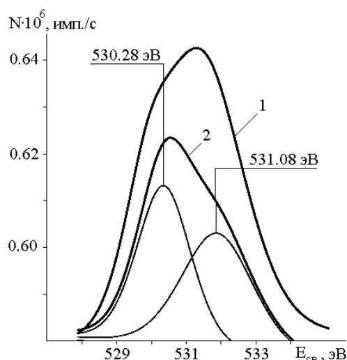
Рисунок 2. Профиль пика 1s О с поверхности Ag после выдержки в течение 2 час. в паровой фазе при 1073 К (1) и через 20 с ионного травления (2).
