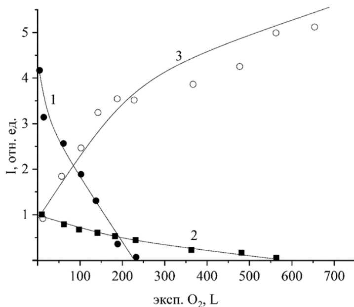
Рис. 6. Зависимости интенсивностей пиков объемных плазмонов (кривая 1 – пик Е, кривая 2 – пик D) и оже-линии KLL кислорода (кривая 3) от времени экспозиции поверхности индия в среде кислорода (0-1000 L).
