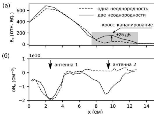
Рис. 3. Поперечное распределение амплитуды свистовой волны в плазме с одной и с двумя неоднородностями (а), формируемыми за счет ВЧ-нагрева, б – поперечное распределение концентрации плазмы; положения антенн указаны стрелками. Источником свистовой волны является антенна, формирующая первую неоднородность. Плотность невозмущенной плазмы N_e = 10^{11} \text{ см}^{-3} , магнитное поле B_0 = 180 \text{ Гс} ; частота пробной волны f = 160 \text{ МГц} , вторая неоднородность формируется излучением с частотой 75 \text{ МГц} . Результаты получены на расстоянии z = 30 \text{ см} от антенн
